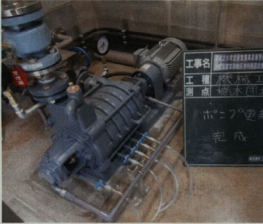
橋木団地 揚水機交換:完成
