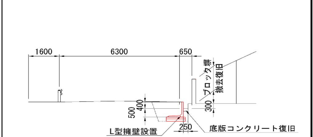
至宇治田原町 標準横断面図
