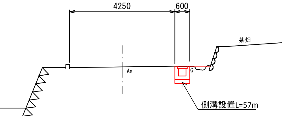
標準断面図
