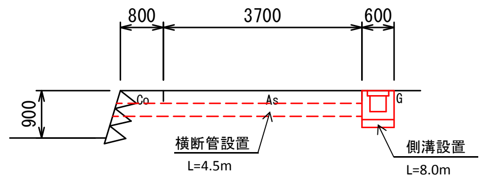
標準断面図
