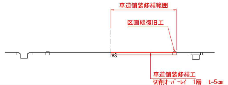
<標準断面図・標準構造図等>
