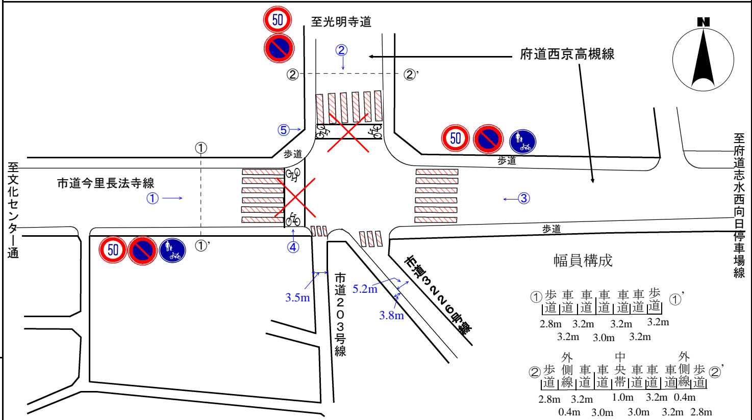
交差点図面
