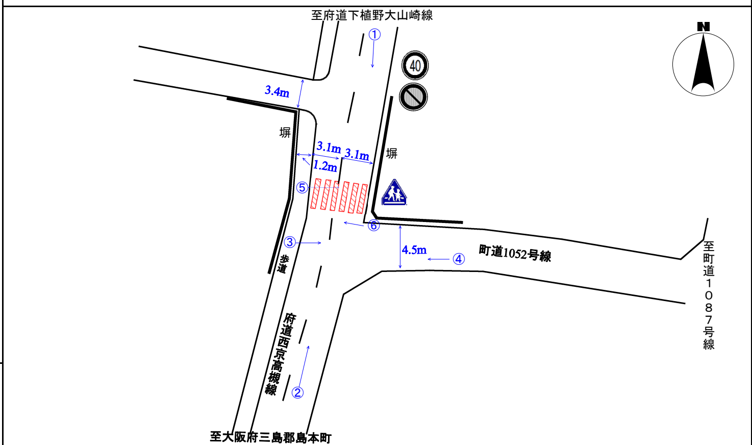
交差点図面
