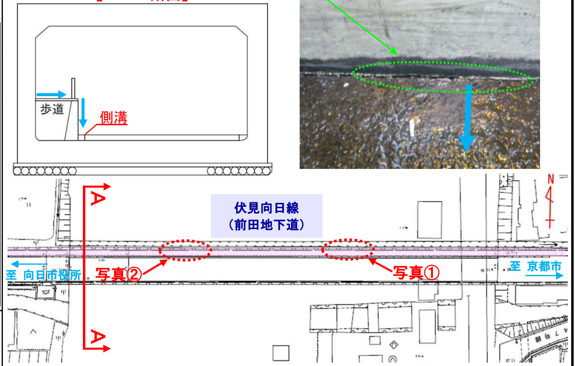
【A-A断面】
