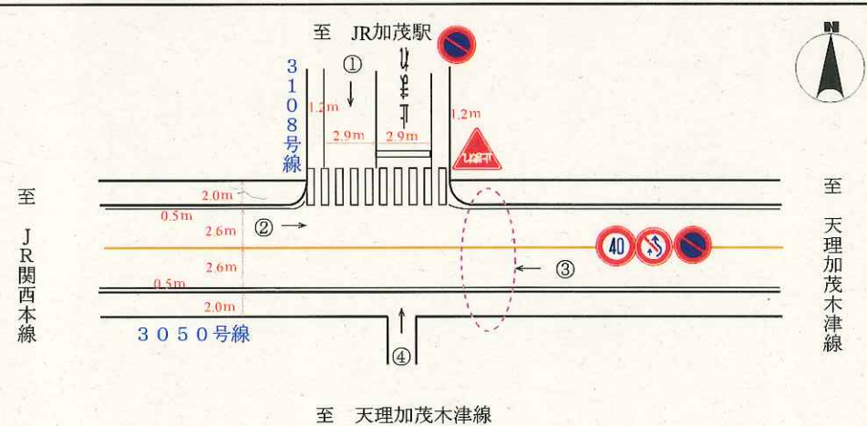
交差点図面
