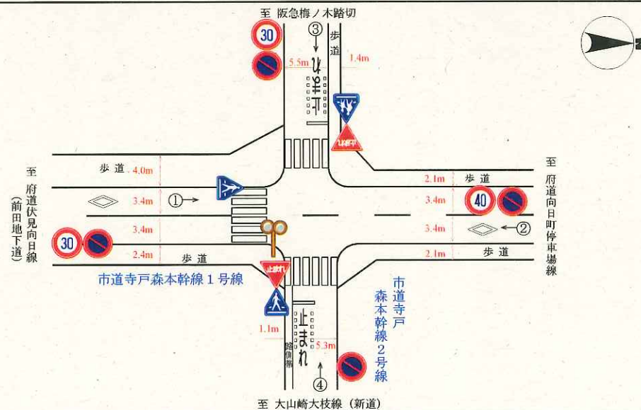
交差点図面
