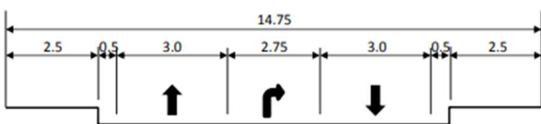
標準横断図
