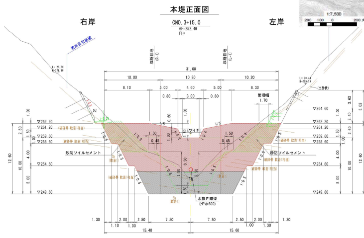
2号堰堤一般構造図
