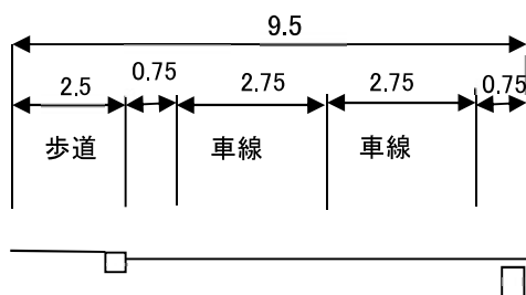
現況幅員5.0m⇒計画幅員9.5m
