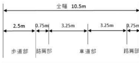
標準断面図
