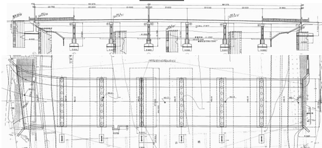
橋梁一般図
