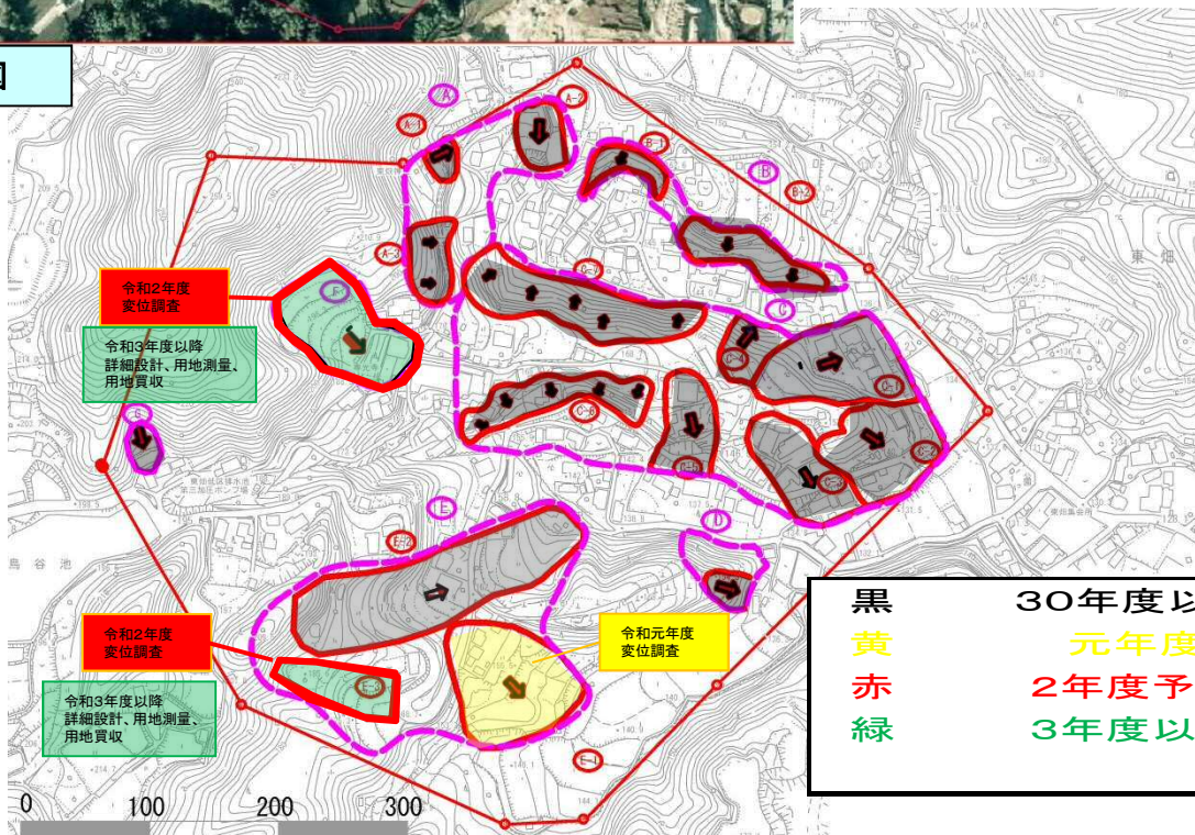
平面図
