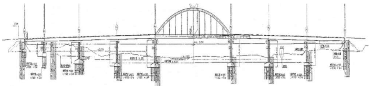
側面図
