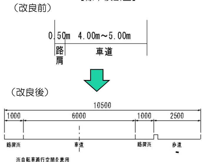
【標準横断図】
