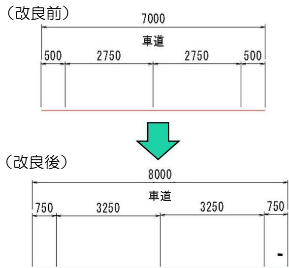
【標準横断図】
