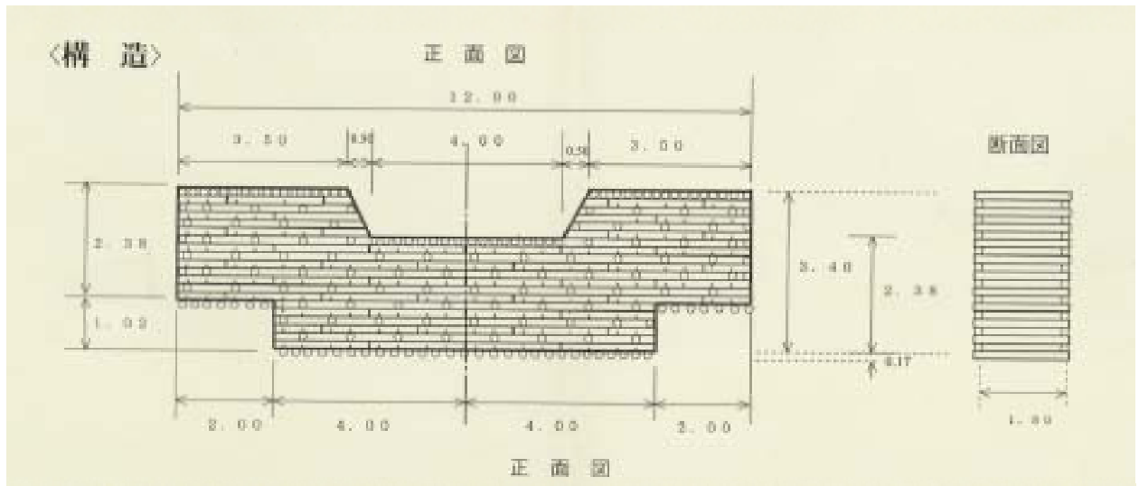
台形型 構造図
