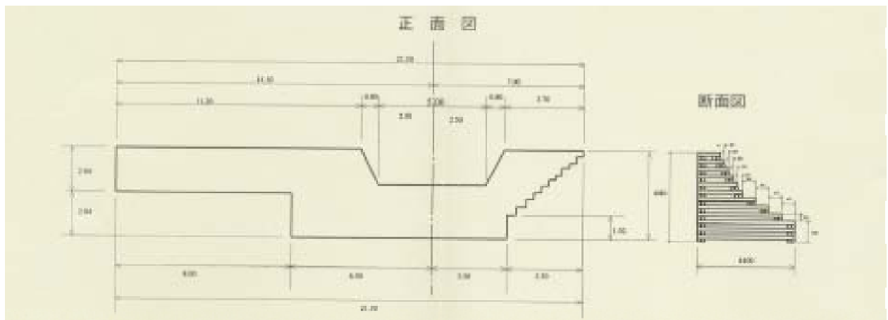
型 構造図
