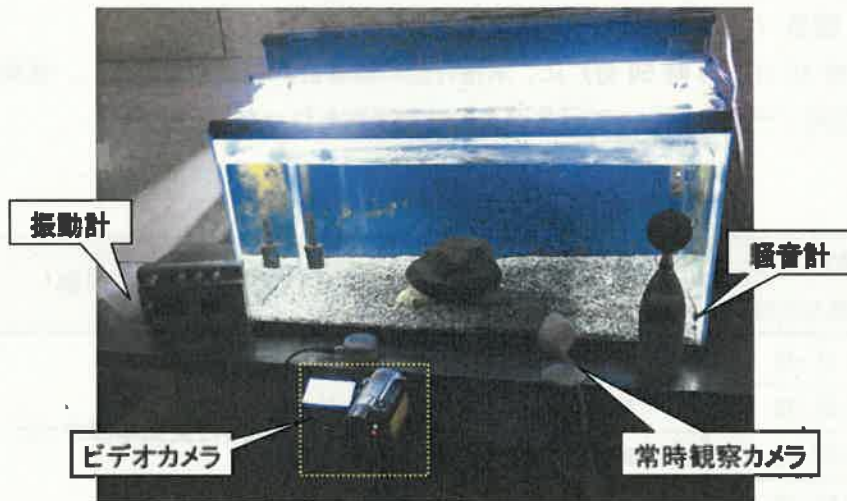
図 10 工事中1回目挙動観察風景（騒音・振動）
