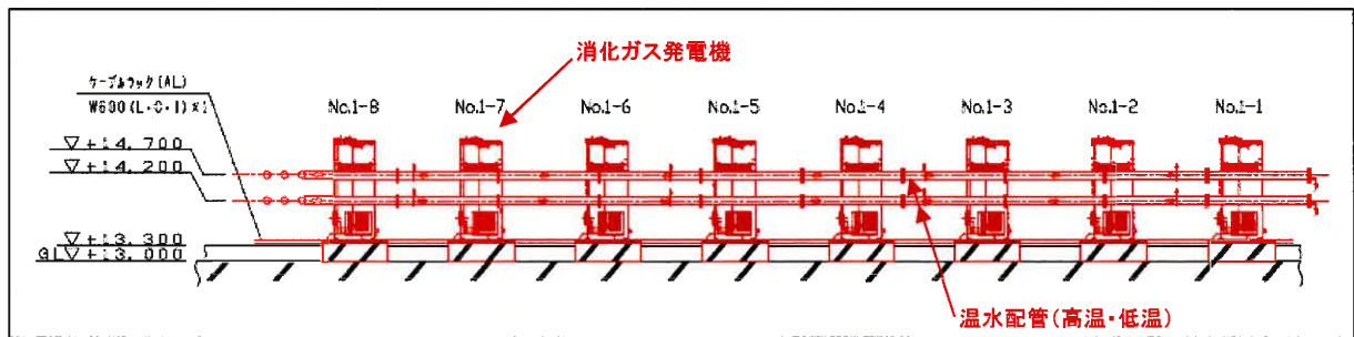
【図4 A-A' 断面図】
