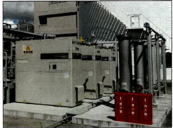
[写真3 同種施設(木津川上流浄化センター)]
