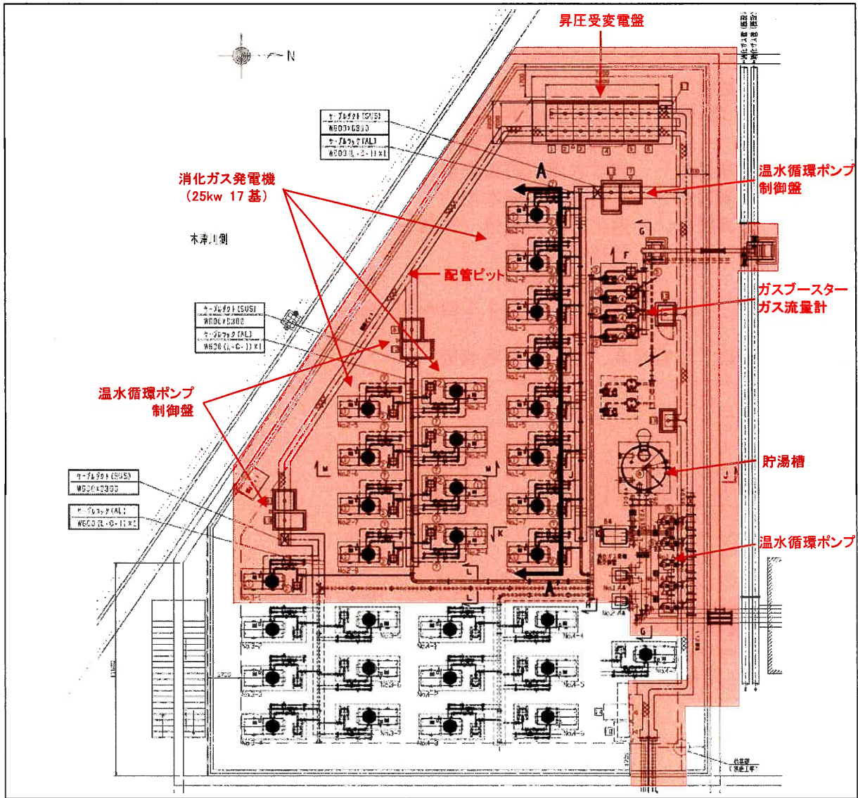
【図3 全体平面図】
