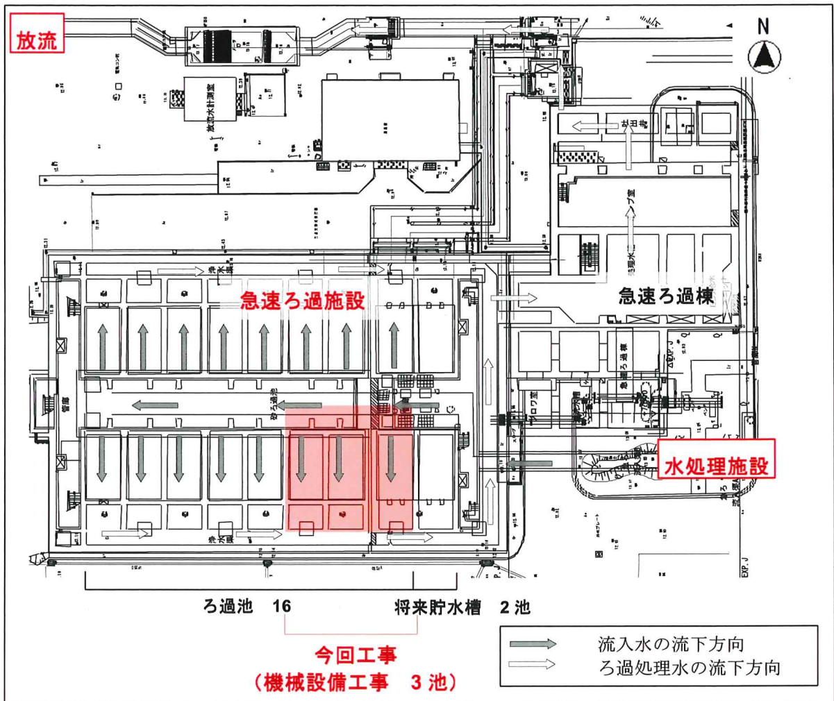
[図3 急速ろ過施設 平面図]
