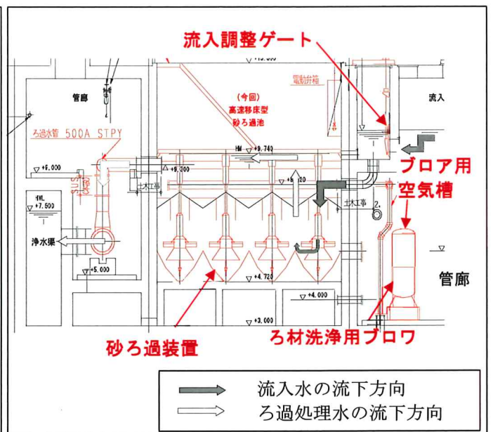
[図5 A-A' 断面図]
