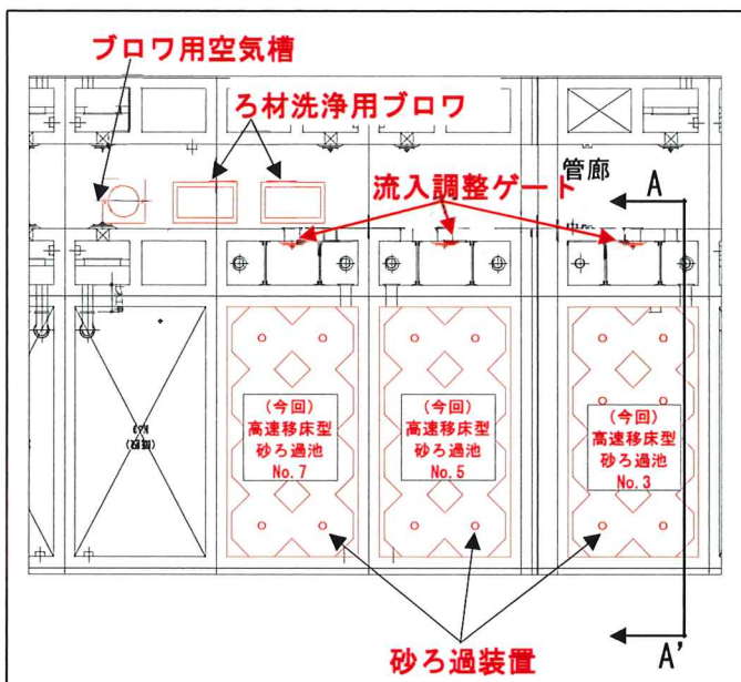
[図4 設備平面図]
