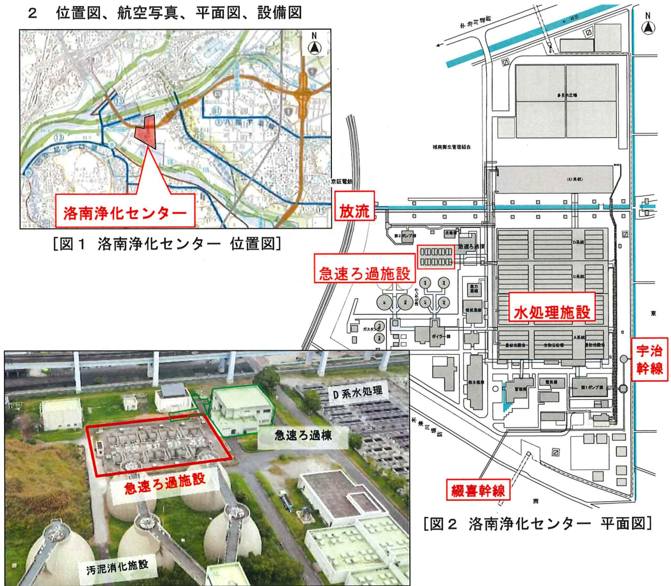
[写真1 急速ろ過施設 施工箇所 航空写真]
