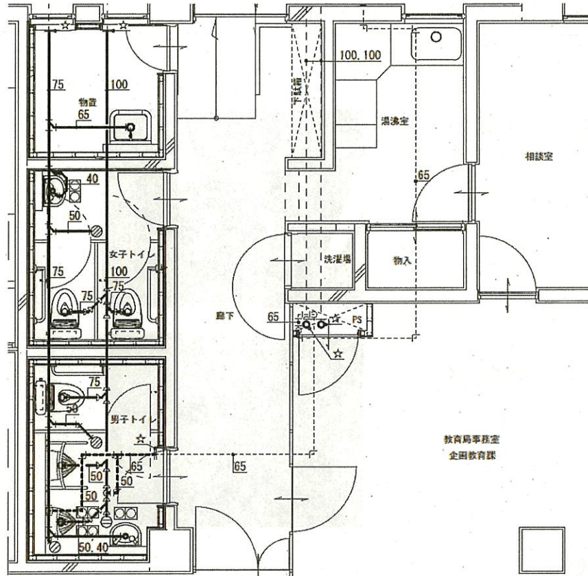
1階改修図
