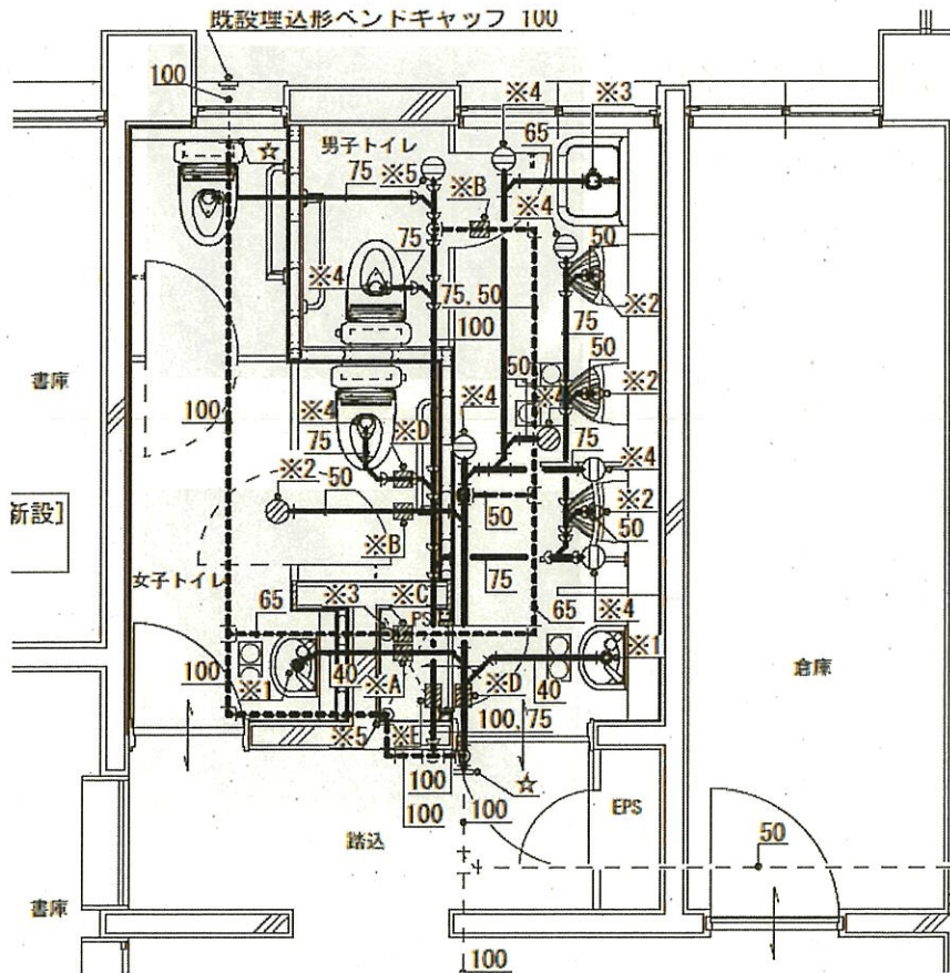
2階改修図
