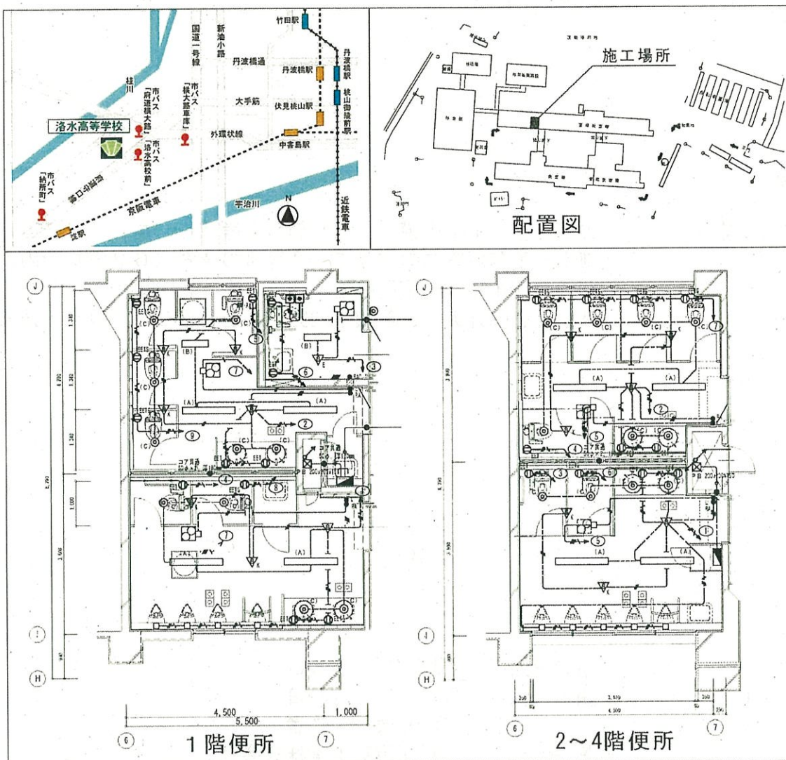
図面は、改修後のもの。LED照明、コンセント、換気扇用電源等の改修。
