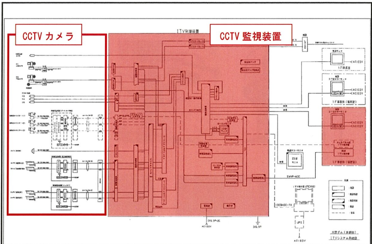
[図3 既存CCTVカメラシステム構成図]
