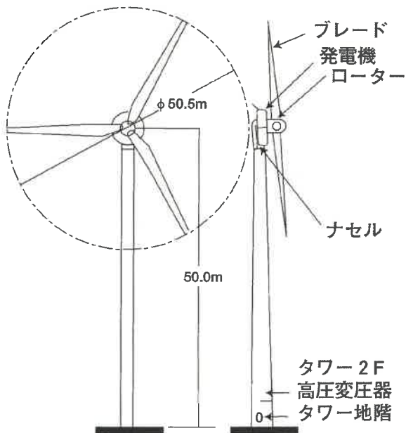
風車の構造図
