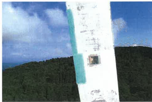
④ ガラス繊維シートにより補強
