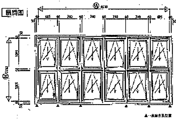
天窓展開図
