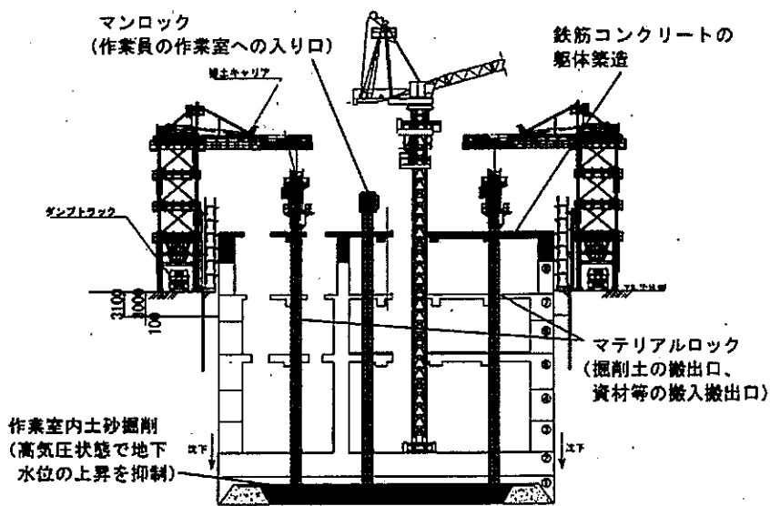
【作業概要横断図】
