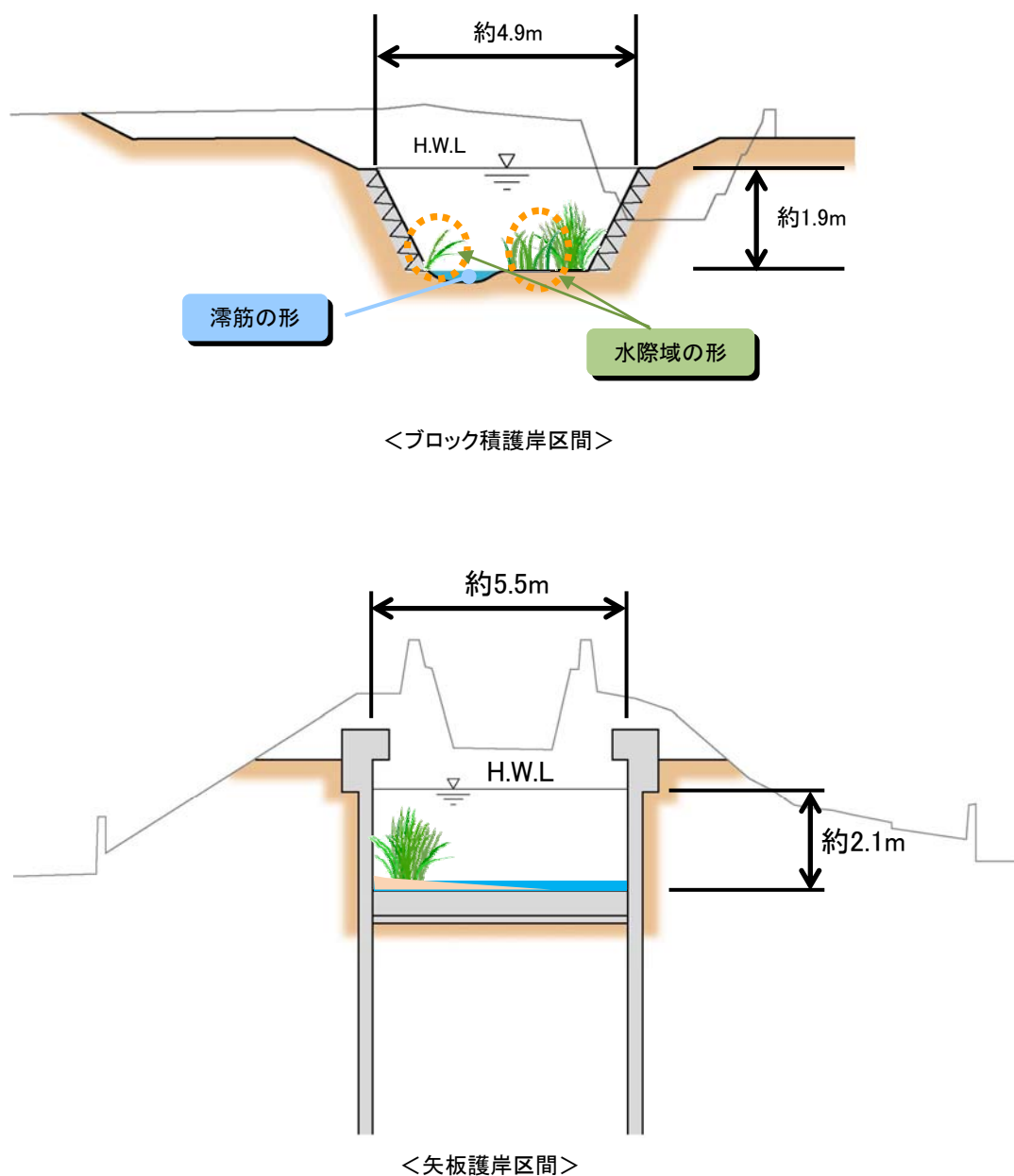
図 2-18 弥陀次郎川標準横断面図
