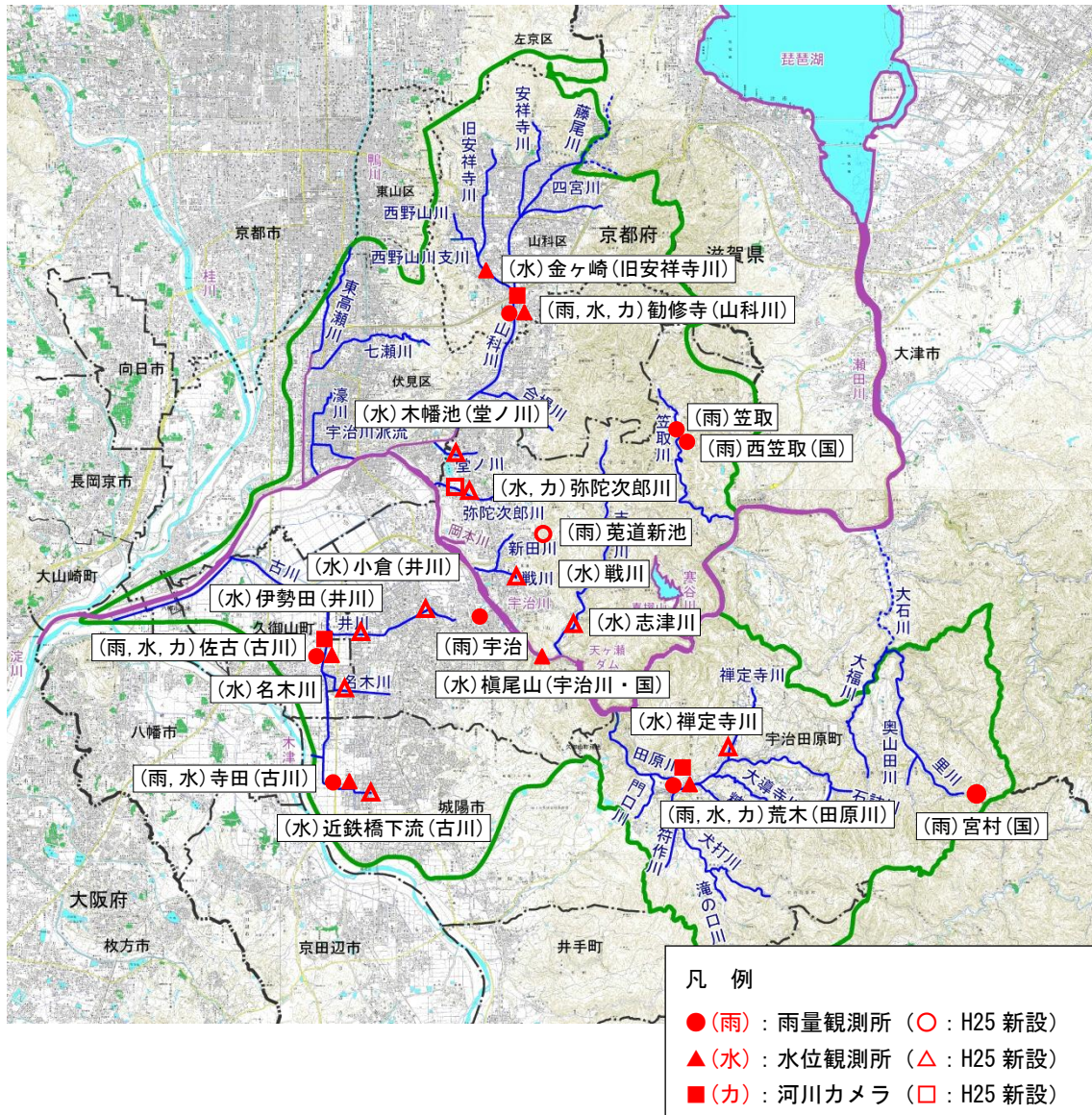
図 3-2 雨量・水位等の観測機器設置状況
