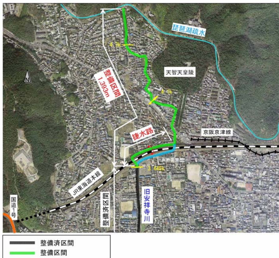
図 2-10 旧安祥寺川の整備区間
