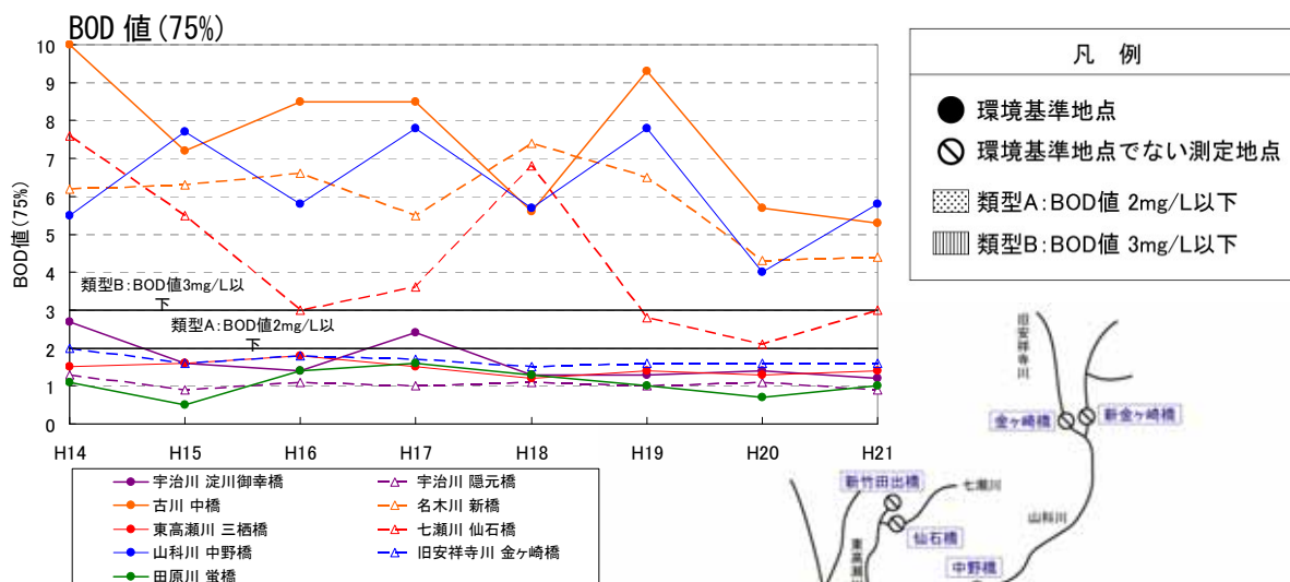
図 1-10 水質の経年変化
