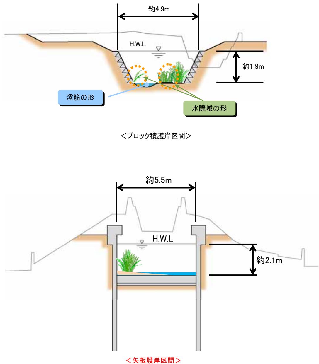
図 2-18 弥陀次郎川標準横断面図
