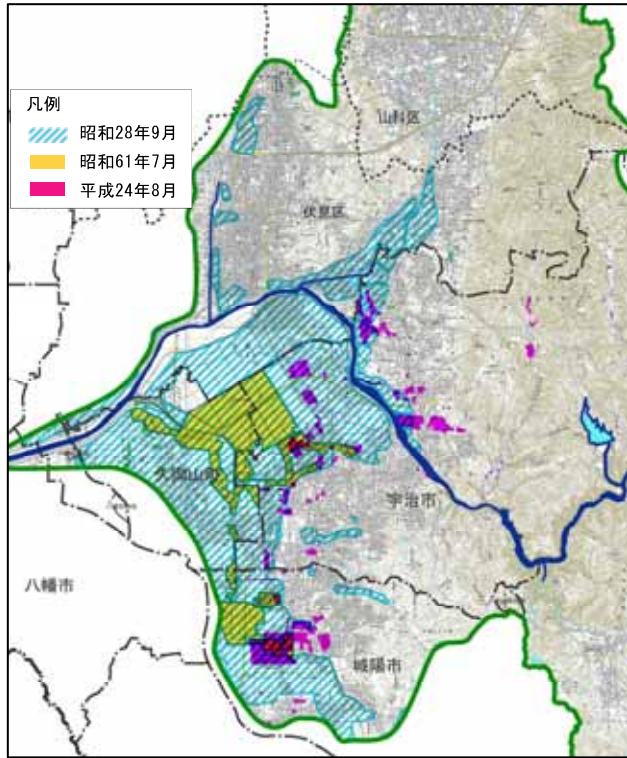
図 1-6 主要洪水の浸水域
