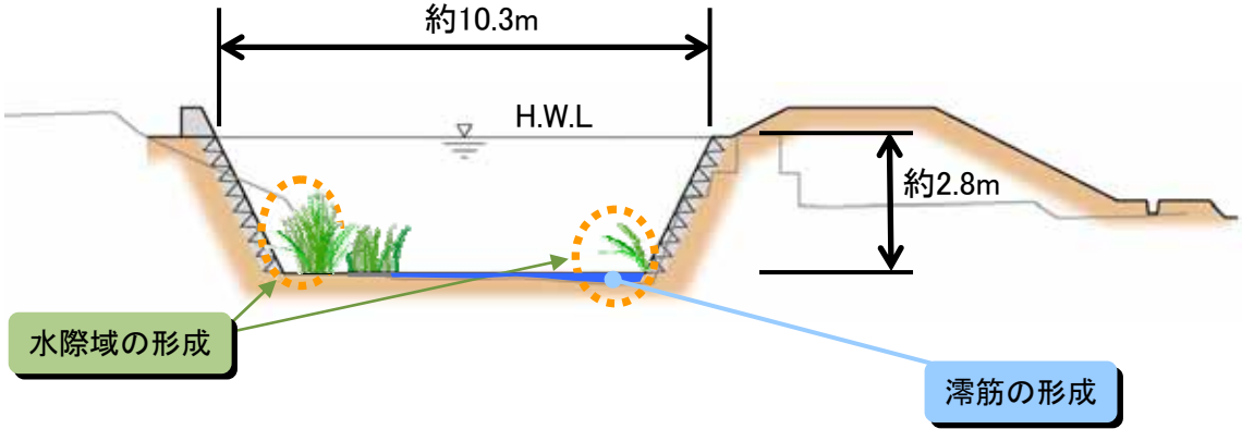
図 2-24 志津川標準横断面図
