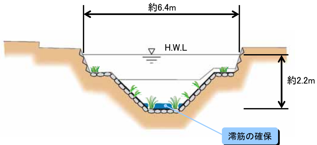
図 2-6 東高瀬川標準横断面図
