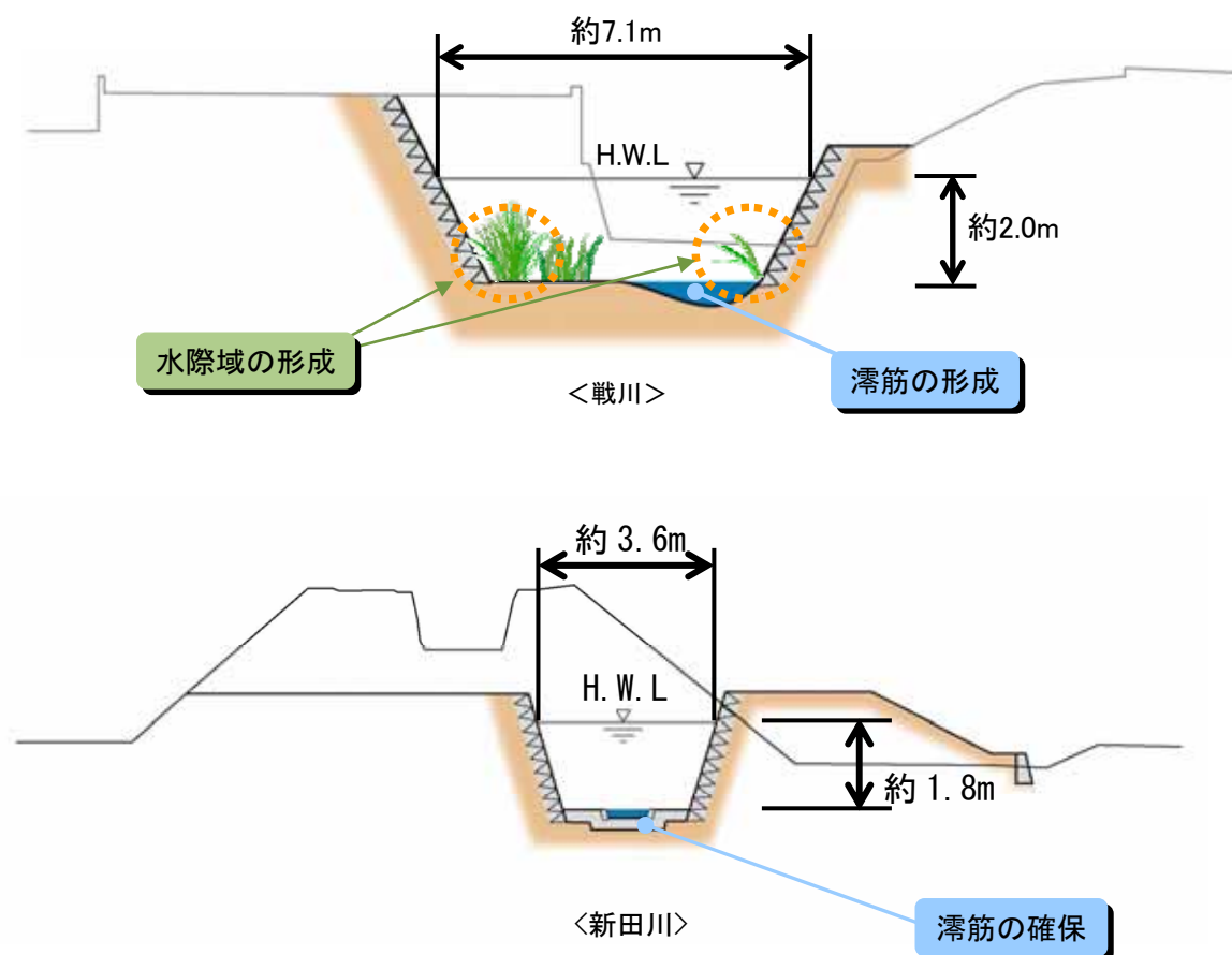
図 2-21 戦川・新田川標準横断面図
