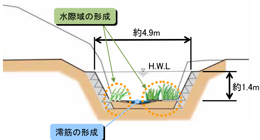
図 2-9 七瀬川標準横断面図
