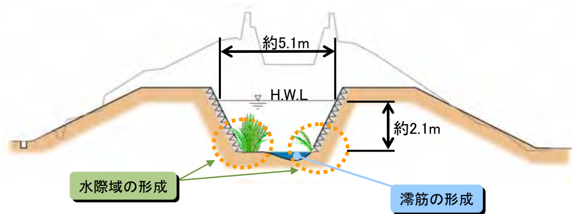
図 2-18 弥陀次郎川標準横断面図
