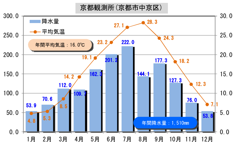
図 1-3 気温と降水量
