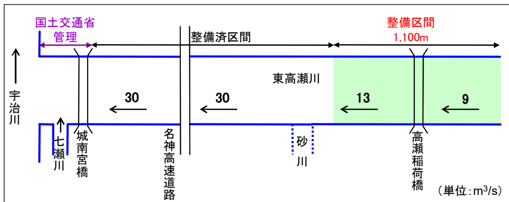
図 2-5 東高瀬川計画流量配分図 (1/10 規模)
