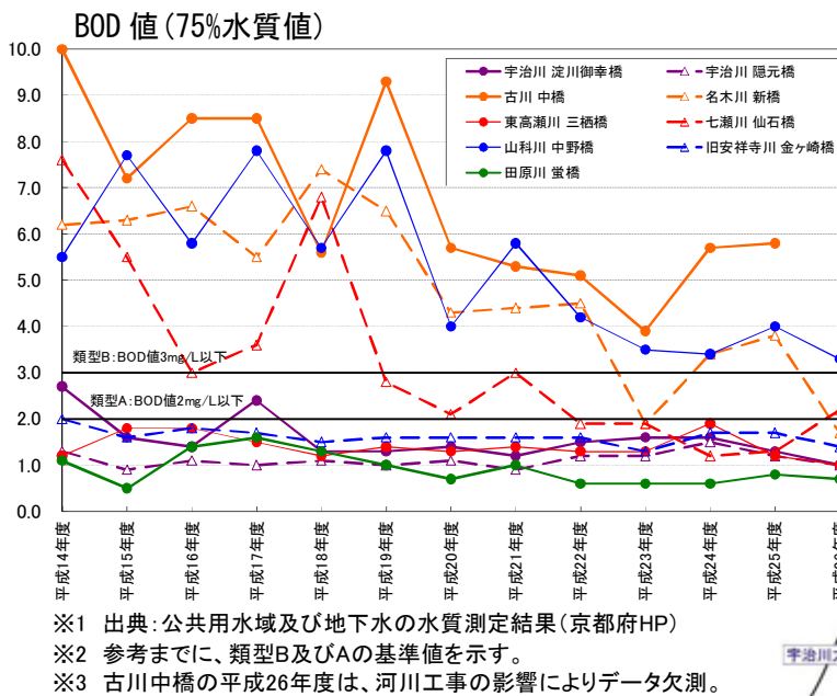
図 1-10 水質の経年変化
