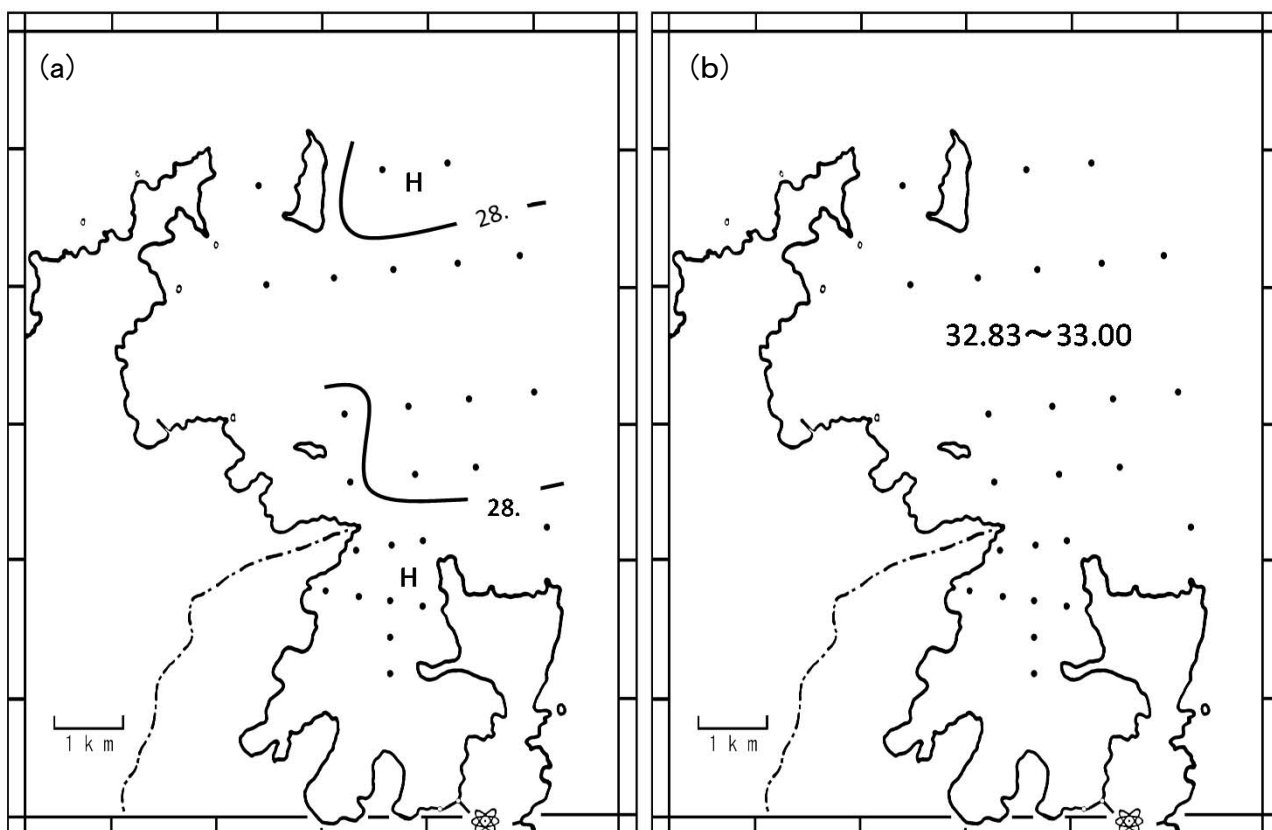
図2-3 表層水温(a)および表層塩分(b)分布図(平成30年8月)
