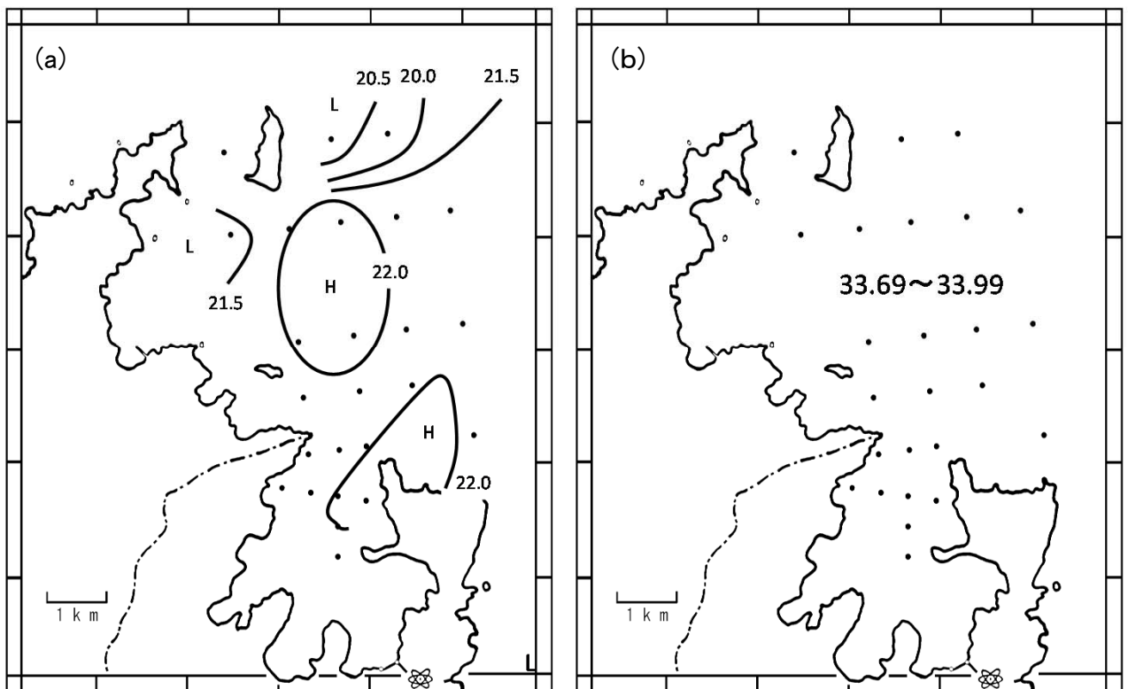
図2-2 表層水温(a)および表層塩分(b)分布図(平成30年6月)
