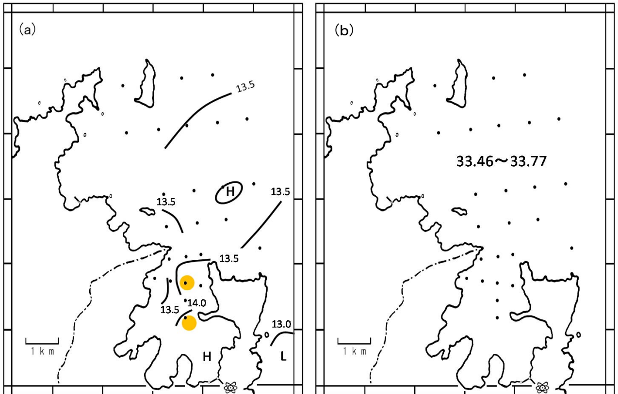
図2-1 表層水温(a)および表層塩分(b)分布図(平成30年4月)
