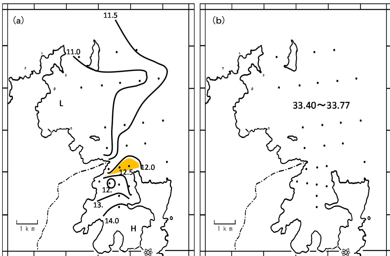
図2-6 表層水温(a)および表層塩分(b)分布図(平成31年2月)
