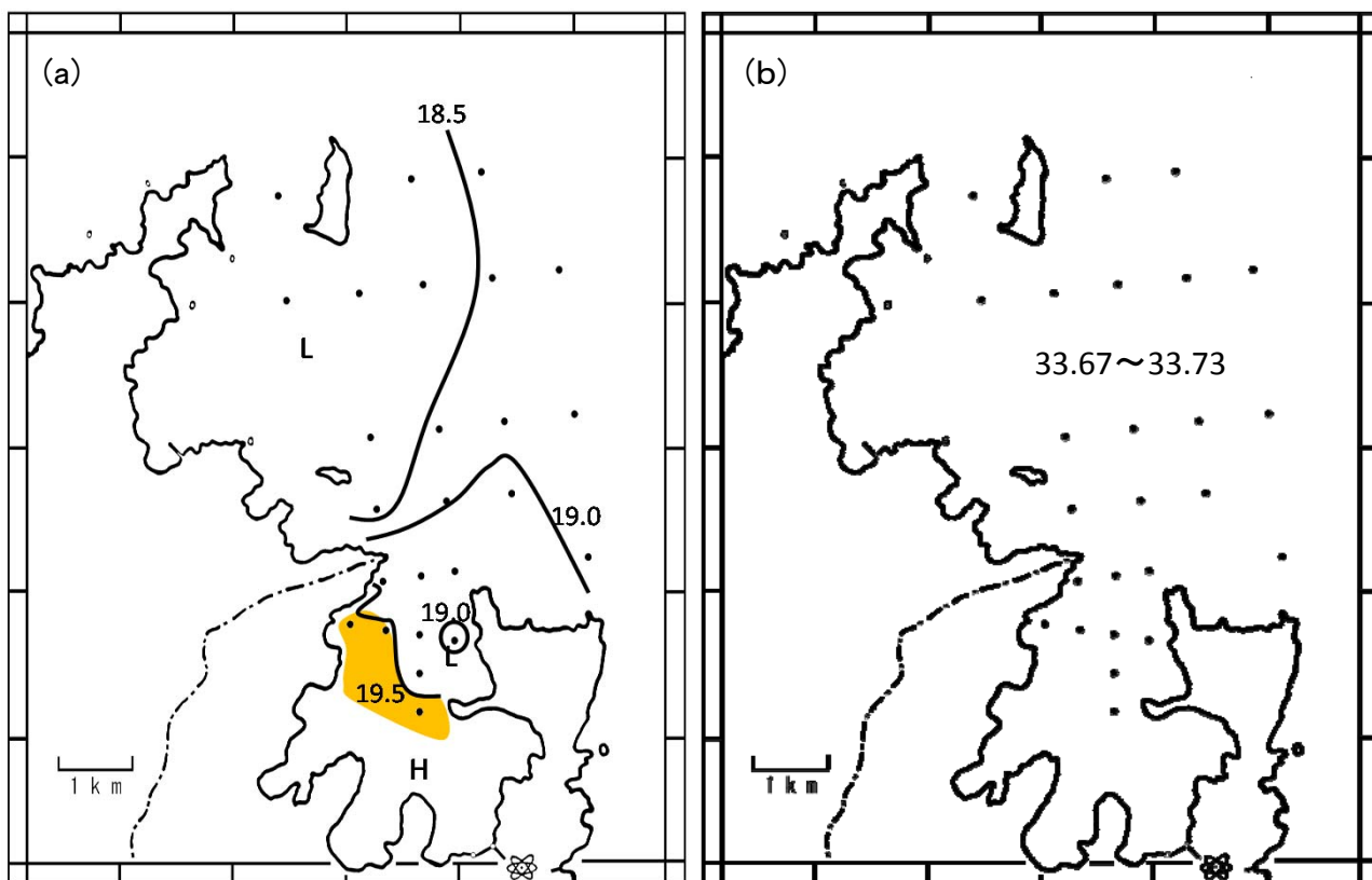
図2-5 表層水温(a)および表層塩分(b)分布図(平成30年12月)
