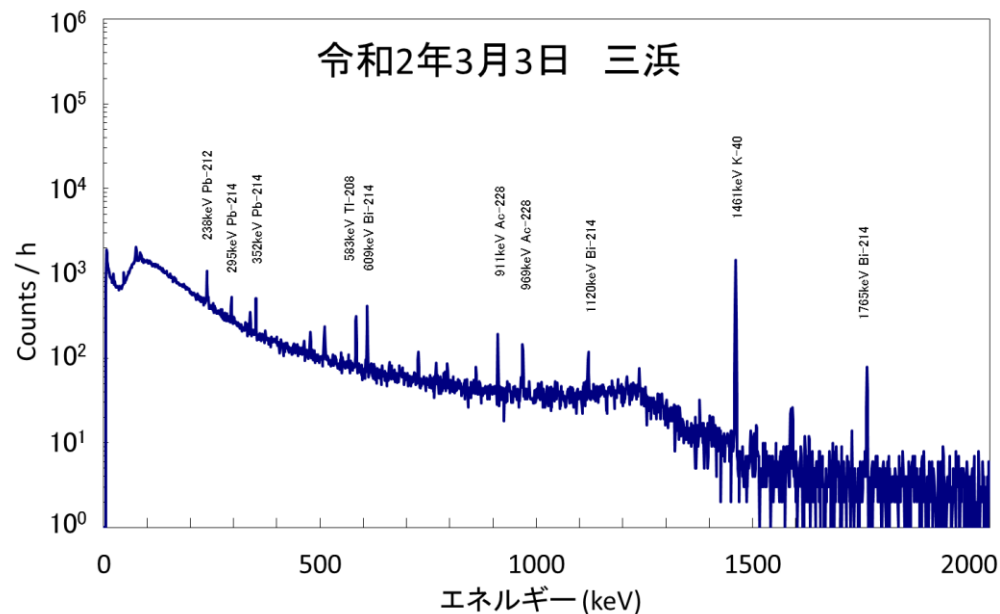
空間ガンマ線スペクトル
