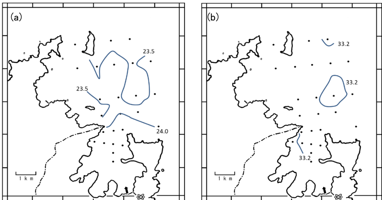
図2-4 表面水温(a)および表面塩分(b)分布図(令和4年10月)
