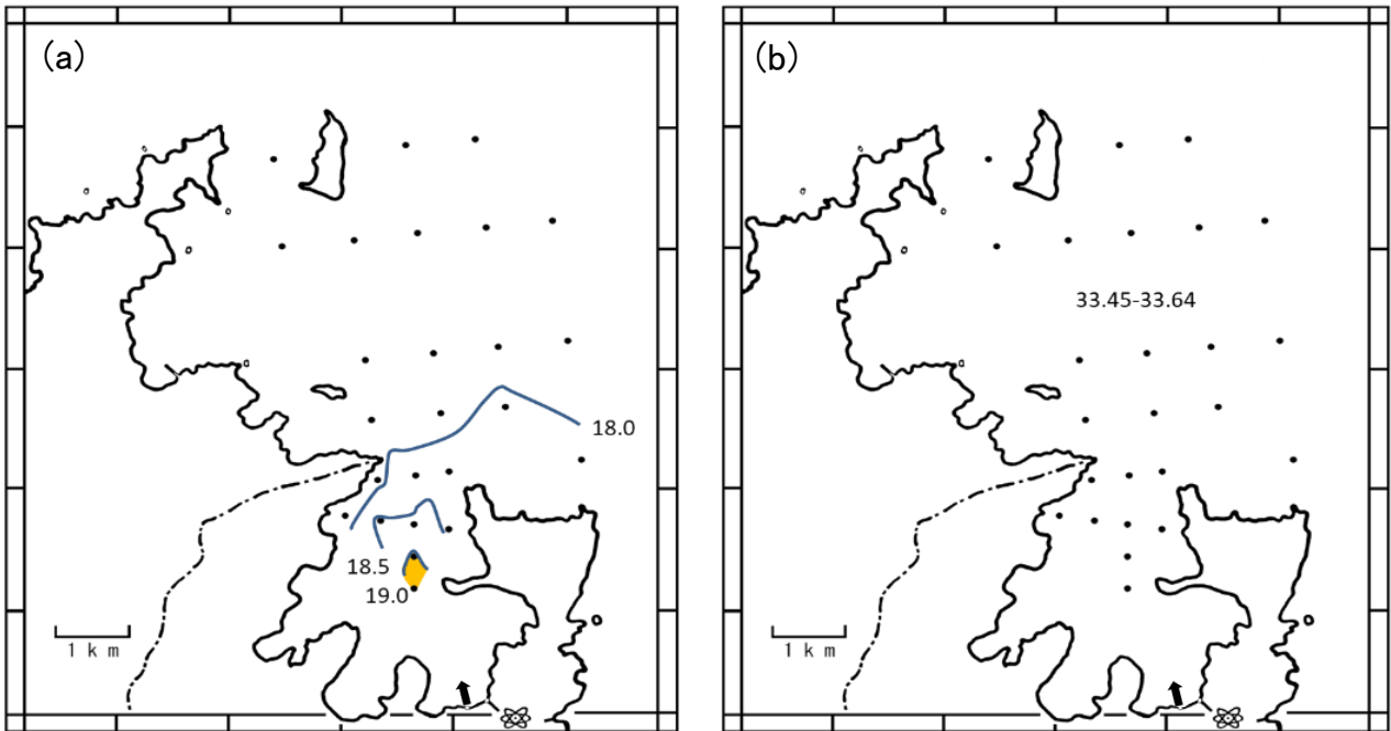
図2-5 表層水温(a)および表層塩分(b)分布図(令和4年12月)
