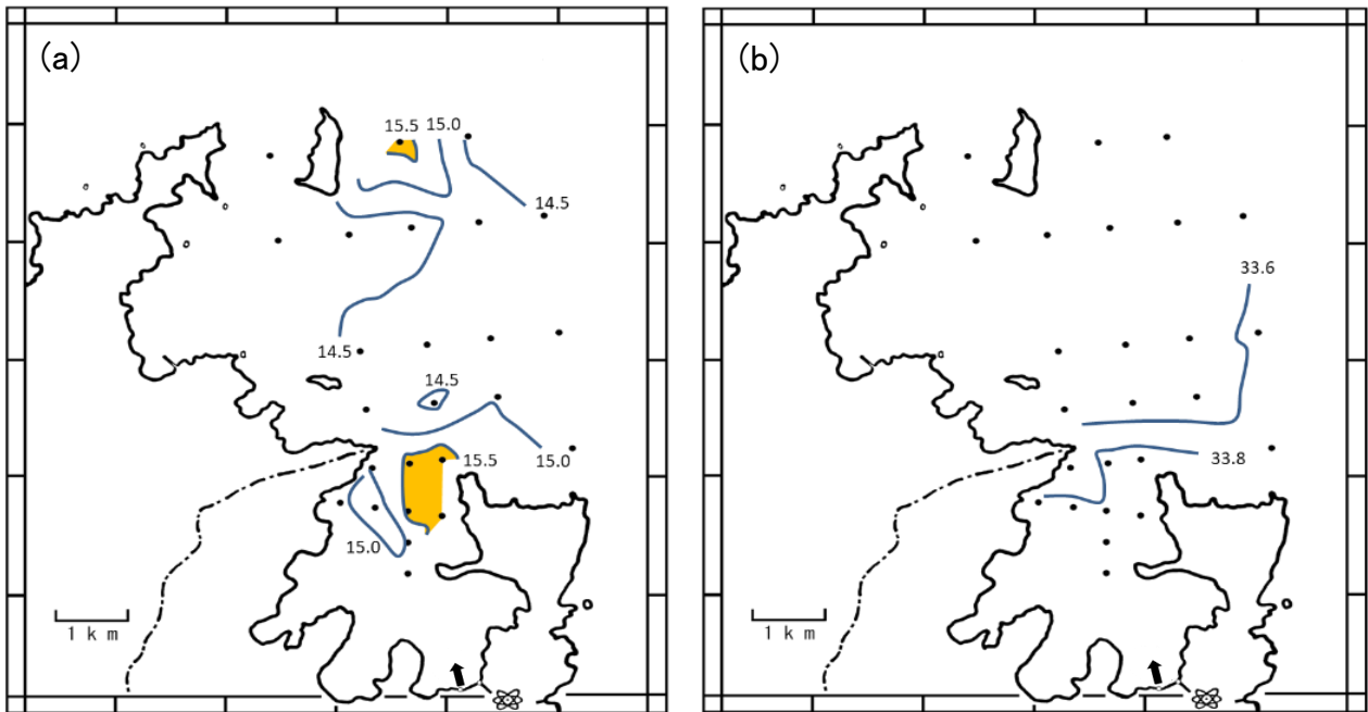
図2-1 表層水温 (a) および表層塩分 (b) 分布図 (令和4年4月)
