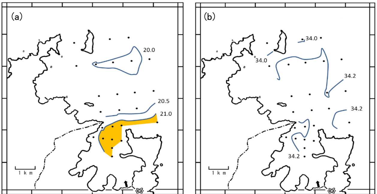
図2-2 表面水温(a)および表面塩分(b)分布図(令和4年6月)
