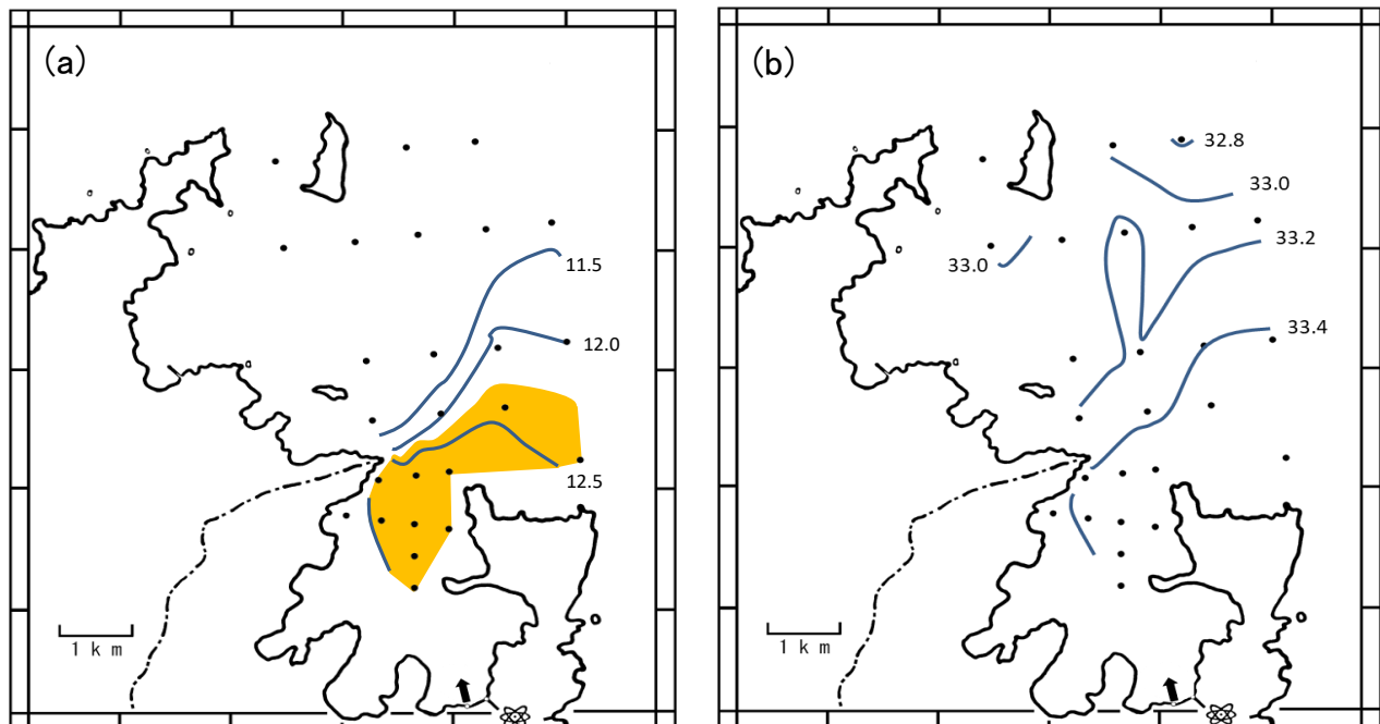
図2-6 表層水温(a)および表層塩分(b)分布図(令和5年2月)
