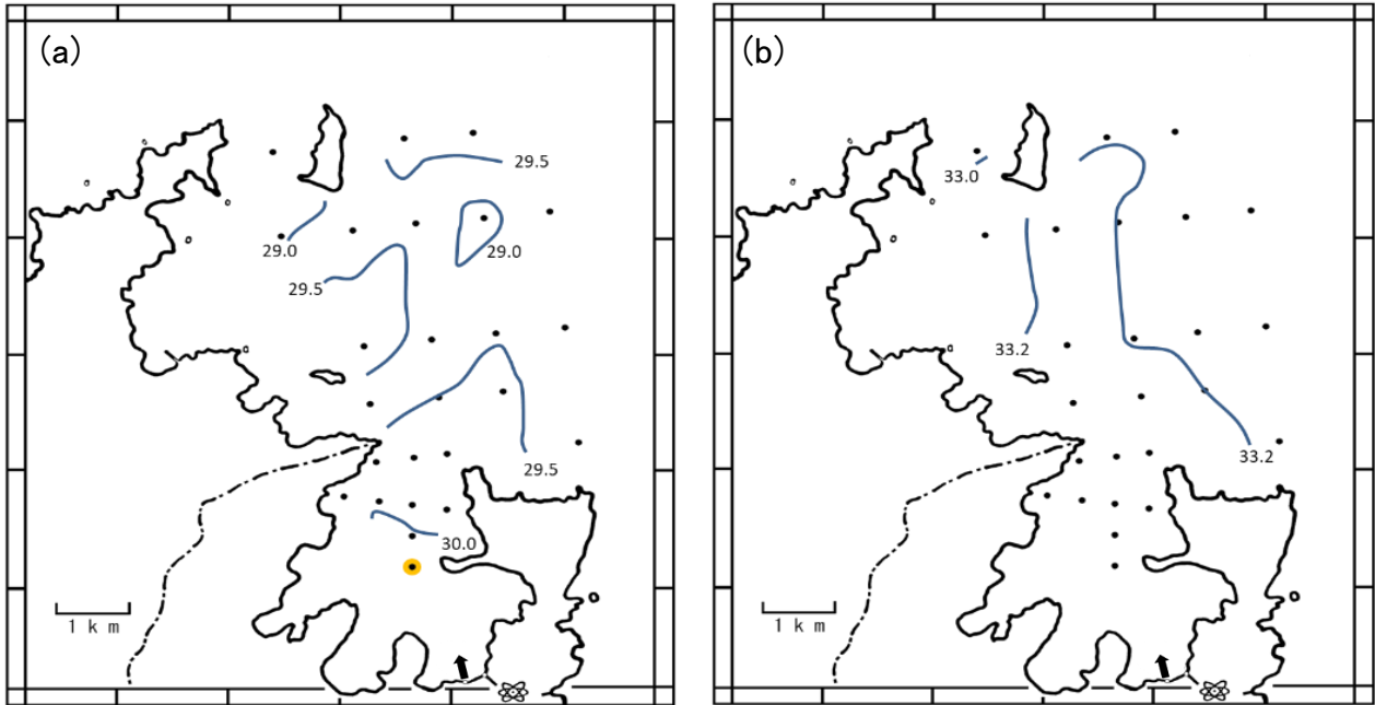
図2-3 表面水温(a)および表面塩分(b)分布図(令和4年8月)
