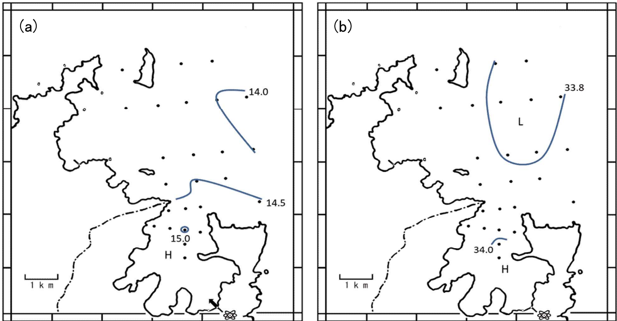
図2-1 表層水温 (a) および表層塩分 (b) 分布図 (令和3年4月)
