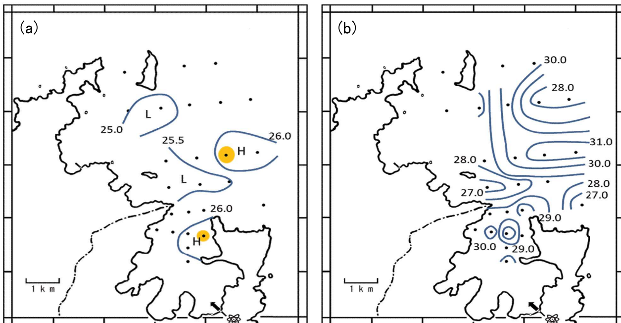
図2-3 表面水温(a)および表面塩分(b)分布図(令和3年8月)
