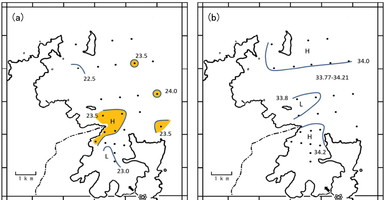
図2-2 表面水温(a)および表面塩分(b)分布図(令和3年6月)
