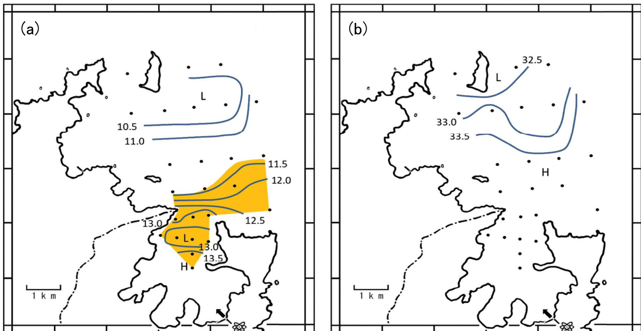
図2-6 表層水温(a)および表層塩分(b)分布図(令和4年2月)
