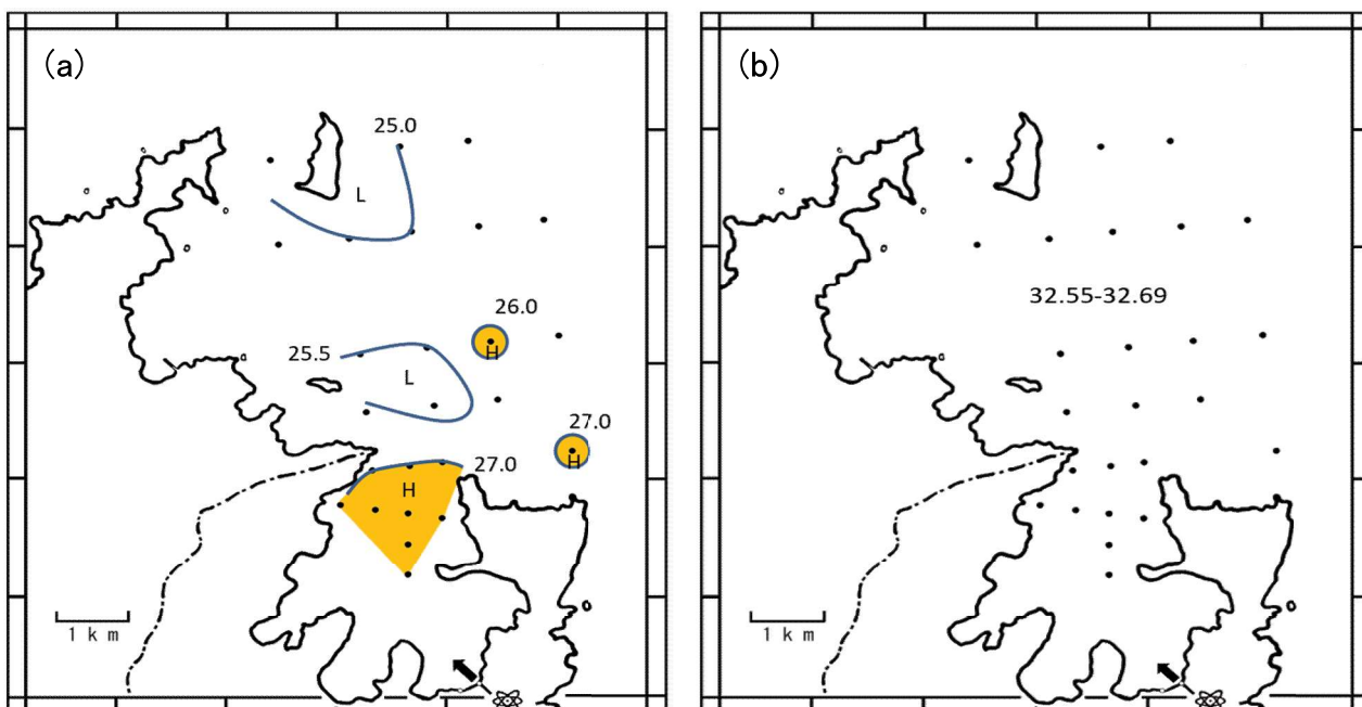
図2-4 表面水温(a)および表面塩分(b)分布図(令和3年10月)
