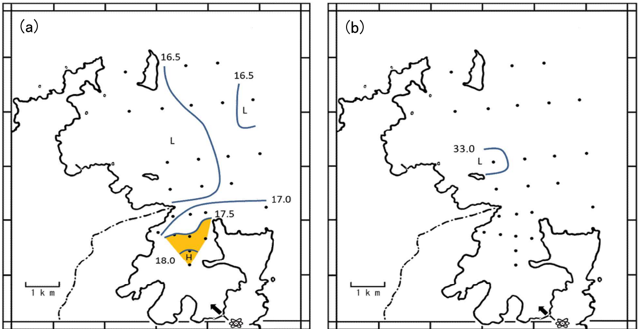
図2-5 表層水温(a)および表層塩分(b)分布図(令和3年12月)
