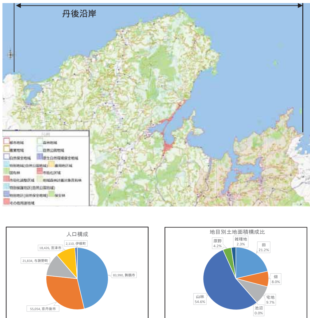
図 1-1-32 土地利用
