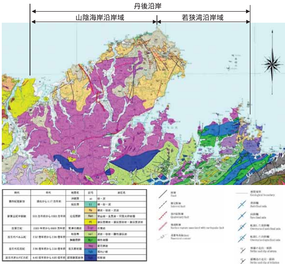
図 1-1-4 広域地質図
