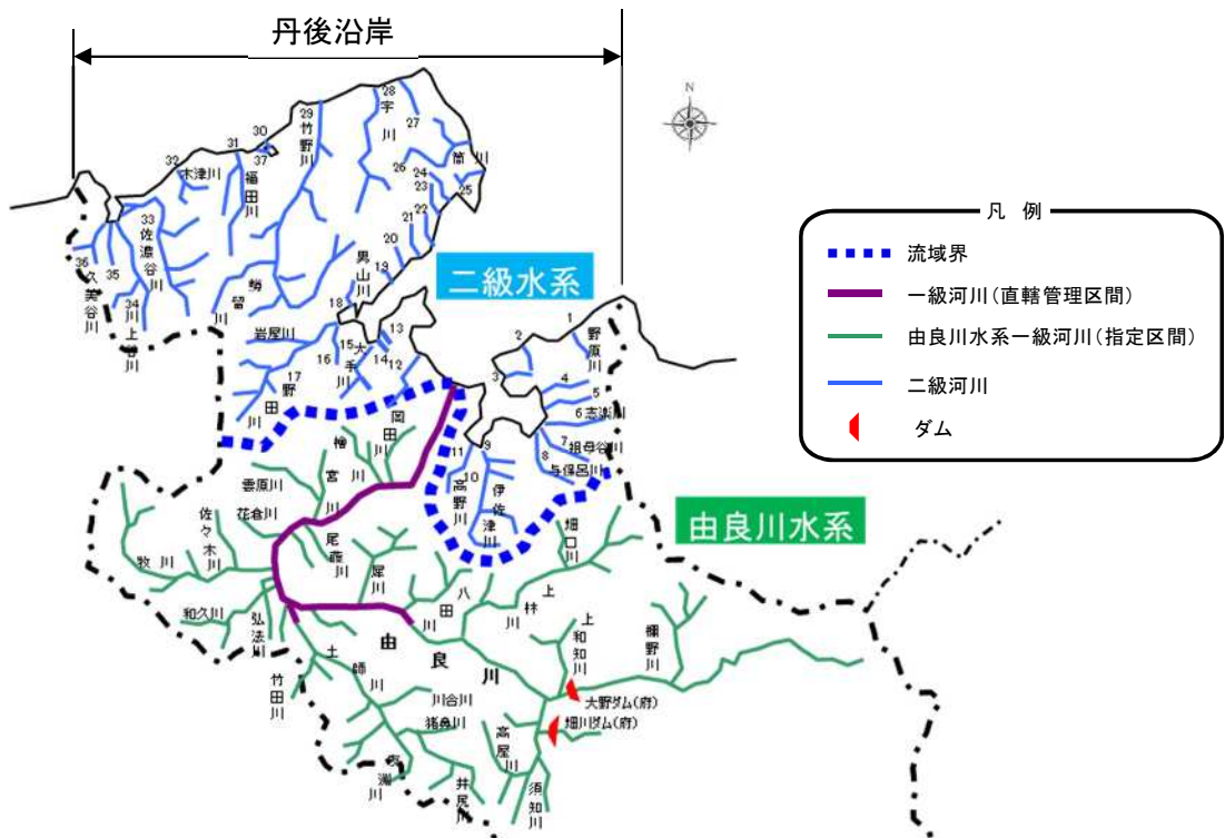
図 1-1-15 丹後沿岸 流入河川位置図
