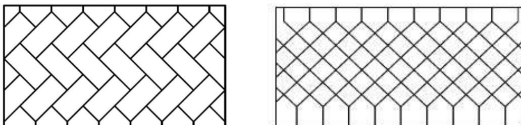
図 3-2-4 谷 積
