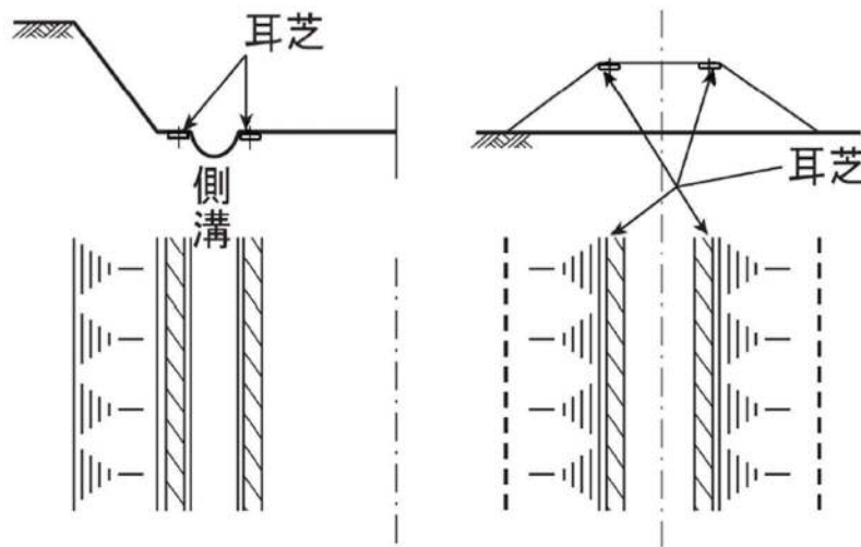
3-2-6 耳 芝
