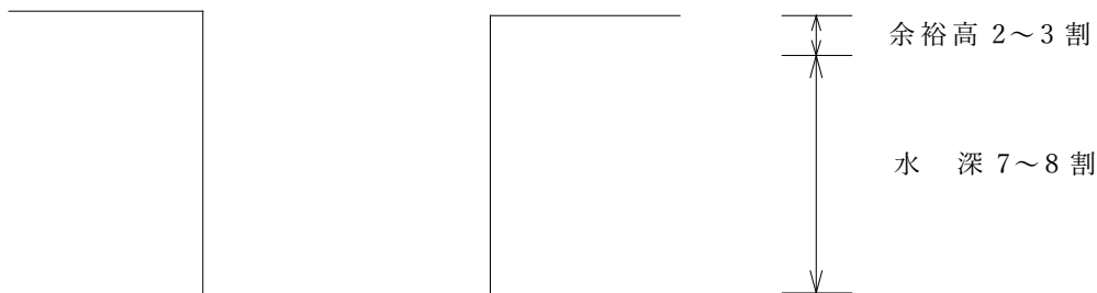
図 1 3 (U字溝、道路側溝)
