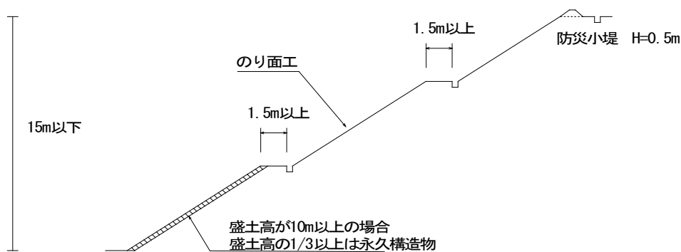
図1 (盛土の標準断面)
