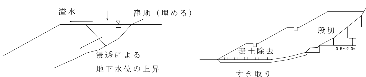
図4 (盛土と地山の接続)
