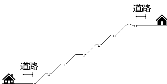
図9 （切土のり面周辺の土地利用上の注意）
