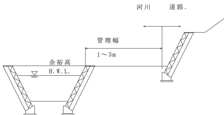
図 1 9 （溪流の付け替えを伴う場合）
