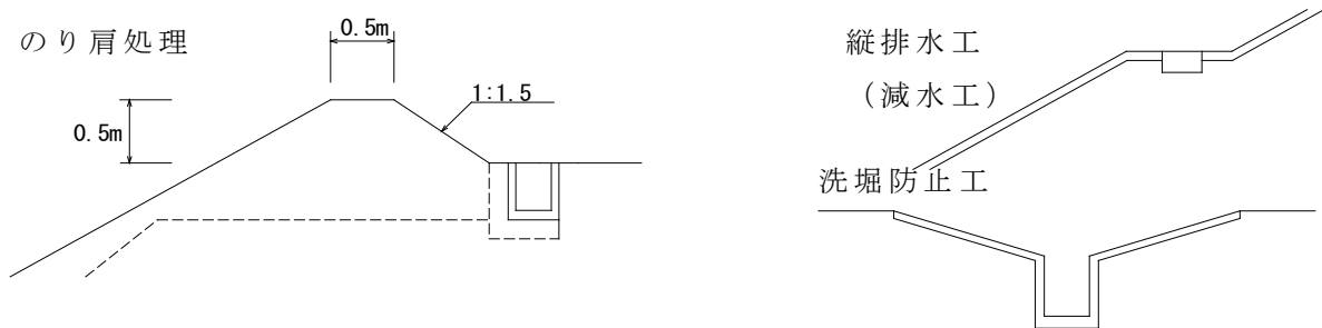
図3 (のり肩処理、縦排水路) 縦排水工
