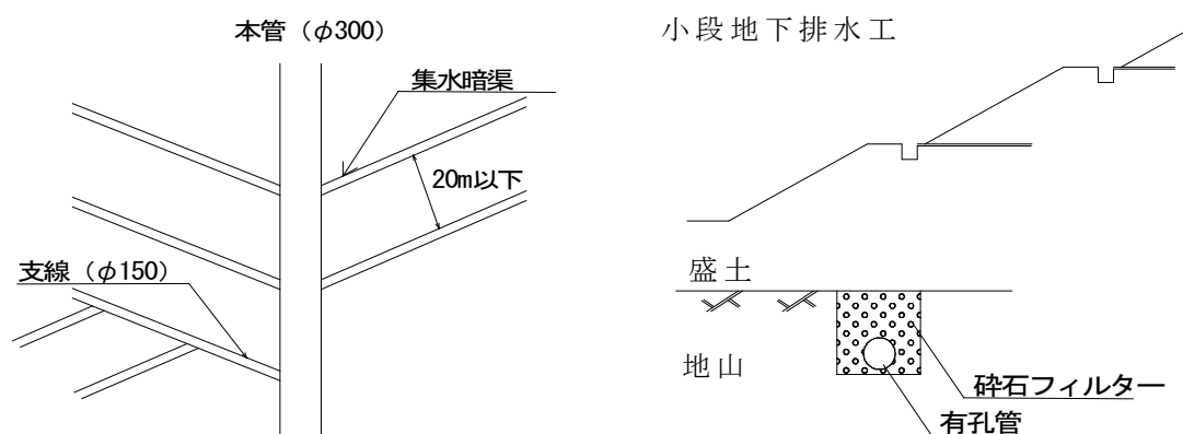
図5 (地下排水工 (暗渠工))
