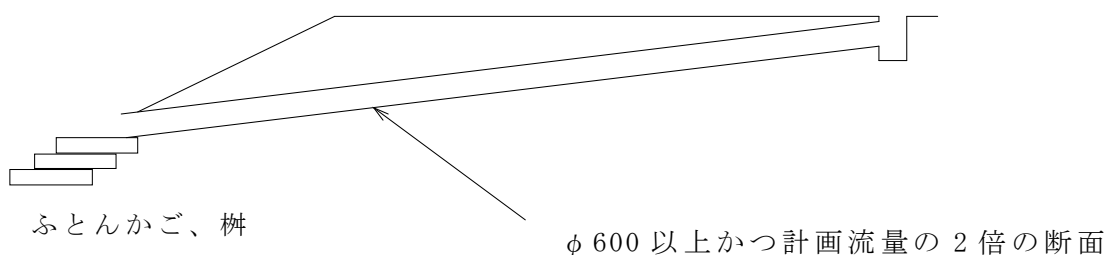
図 1 4 (横断暗渠)
