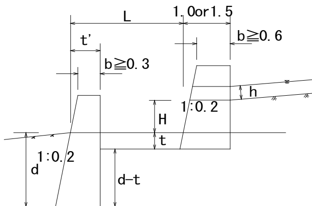
図 1 2 (床固工)
