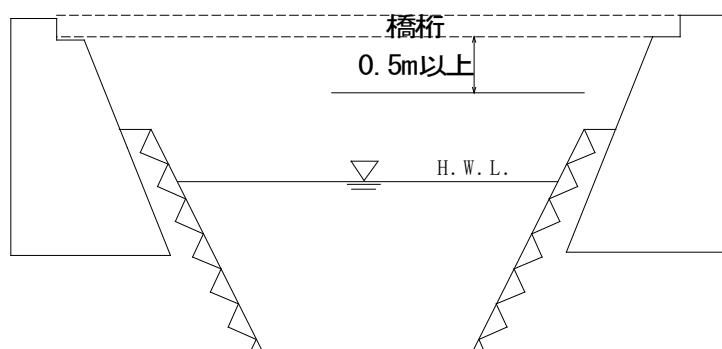
図27 (流域面積0.1km 2 以下の場合)
