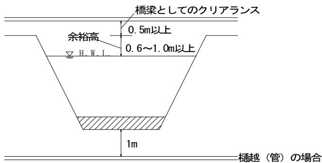
図 29（管類、ケーブル類、架空線類）
