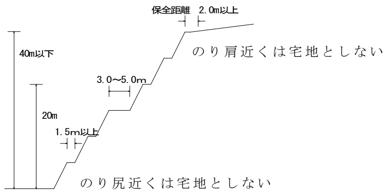
図8 （切土標準断面）
