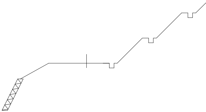
図17 (土工標準断面)
