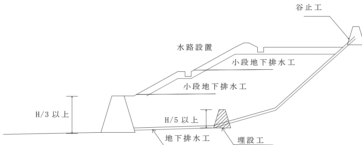
図7 (溪流盛土) 谷止工
