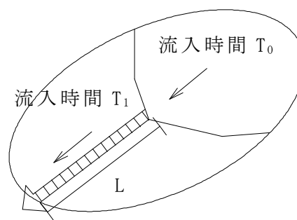
図 10 (洪水到達時間)
