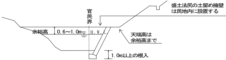
図2 (のり面の末端が流れに接する場合)
