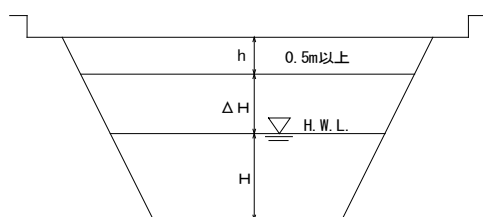
図 2 2（橋梁のクリアランス）
