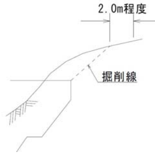
横断面図
