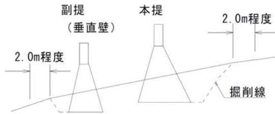
縦断面図
