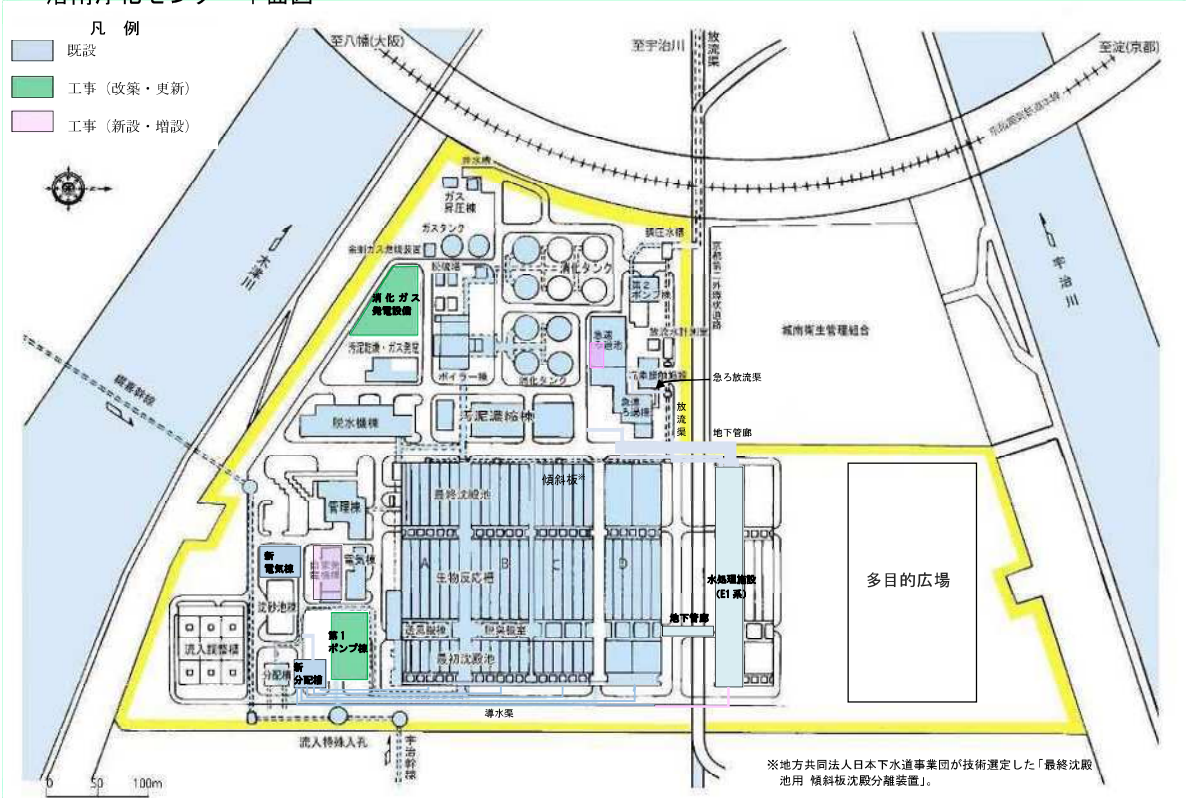
洛南浄化センター平面図
