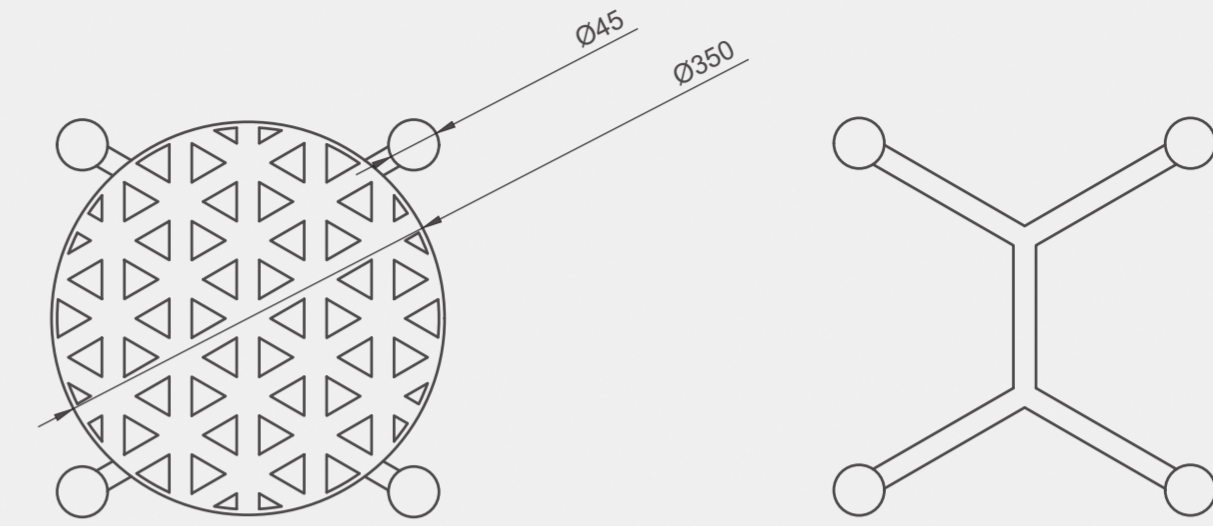
脚上面図
