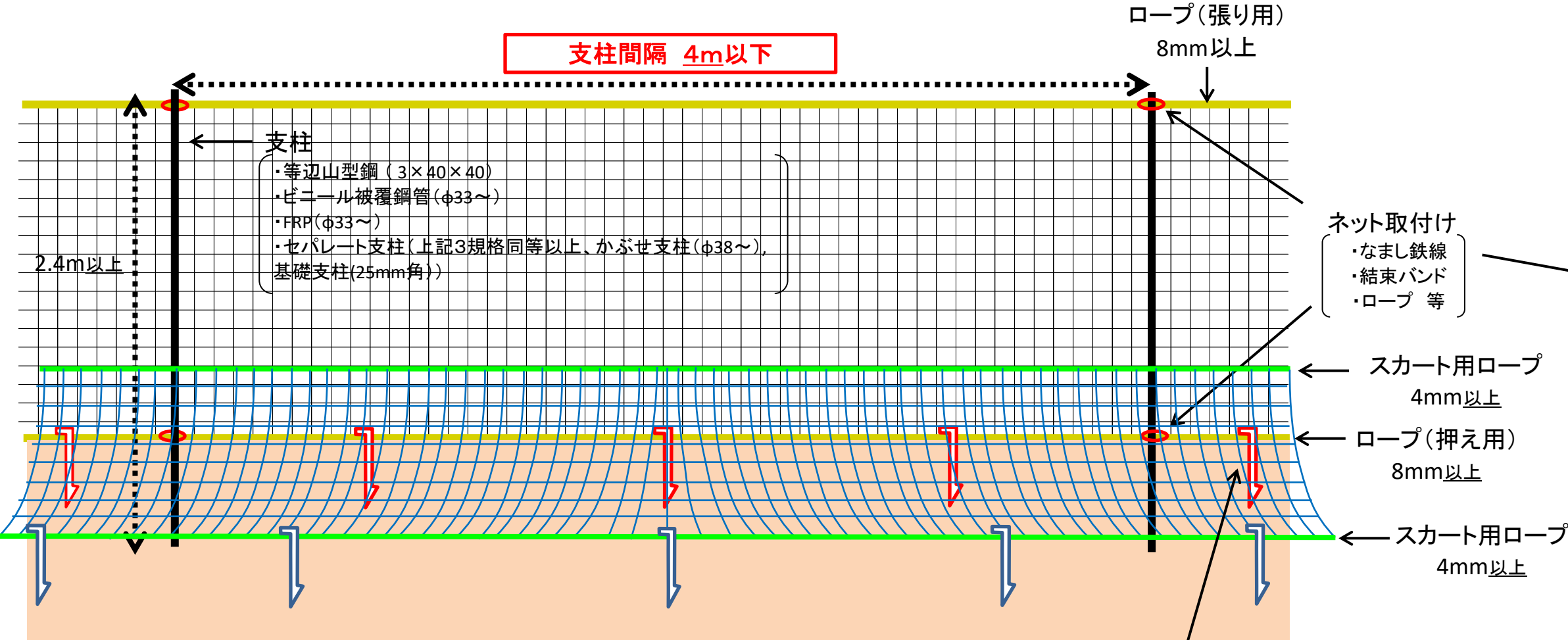
【正面図】
