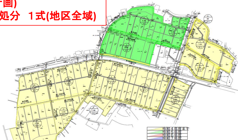
府営農地中間管理機構関連農地整備事業下位田地区計画平面図
