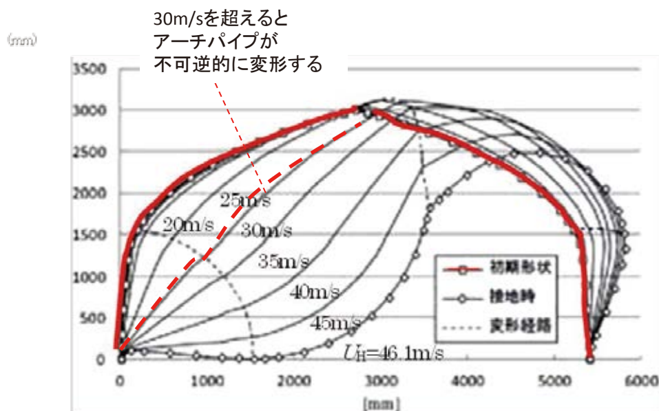
図 ハウス側面からの風に対するアーチパイプの変形
