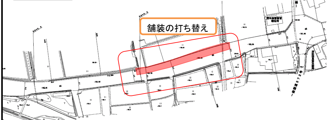
平面図 6 一般地方道大河内口八田線台帳平面図
