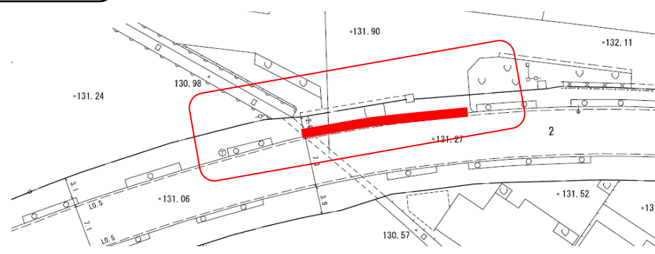
1 主要地方道園部・平屋線台帳平面図
