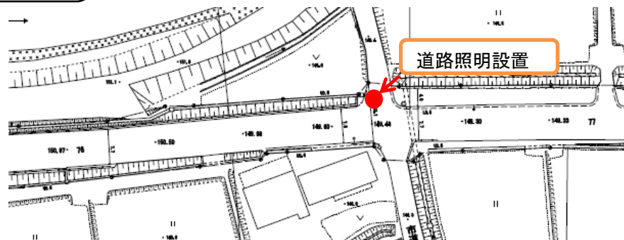
平面図
