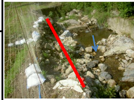
護岸崩壊2
