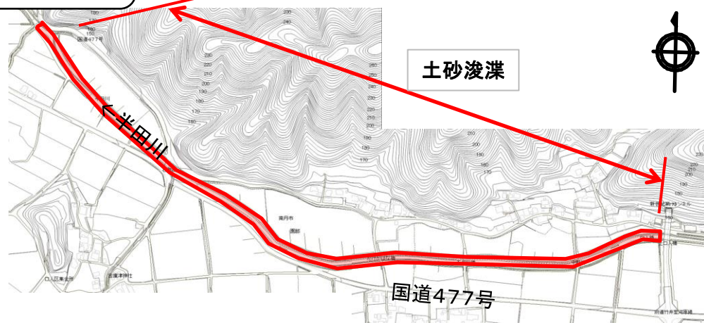
平面図
